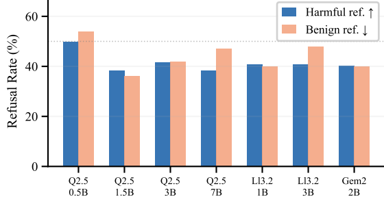
(a) Exp 1: HarmBench — Qwen 2.5 / Llama / Gemma 2
