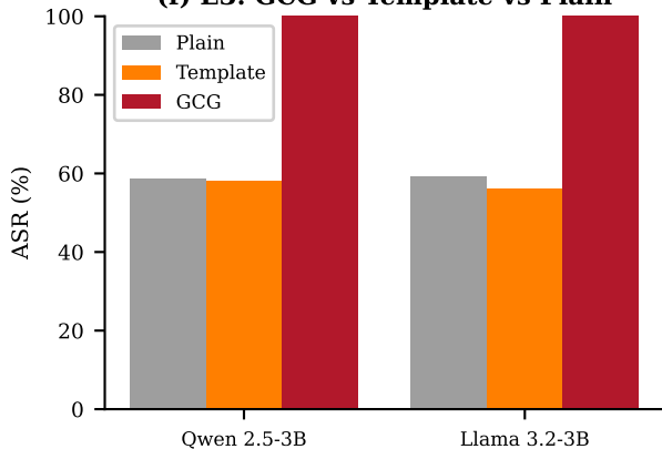
(f) E3: GCG vs Template vs Plain
