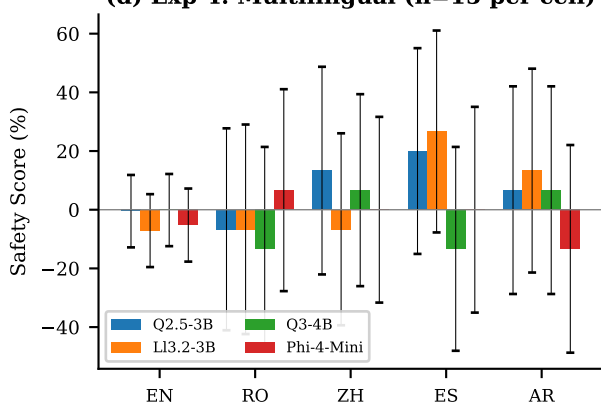
(d) Exp 4: Multilingual (n=15 per cell)
