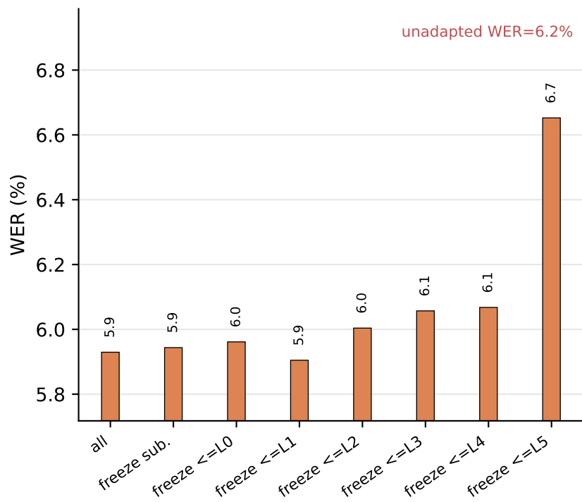
Tedium
