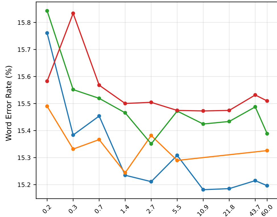
Rev16
