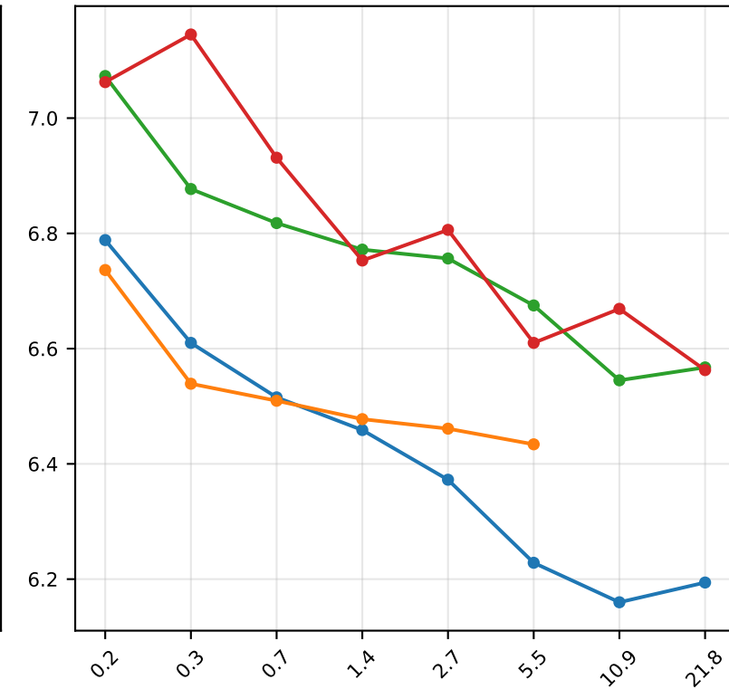
Tedlium
