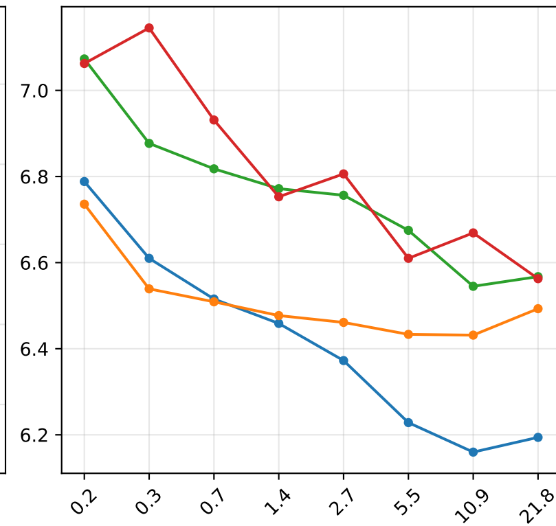
Tedlium
