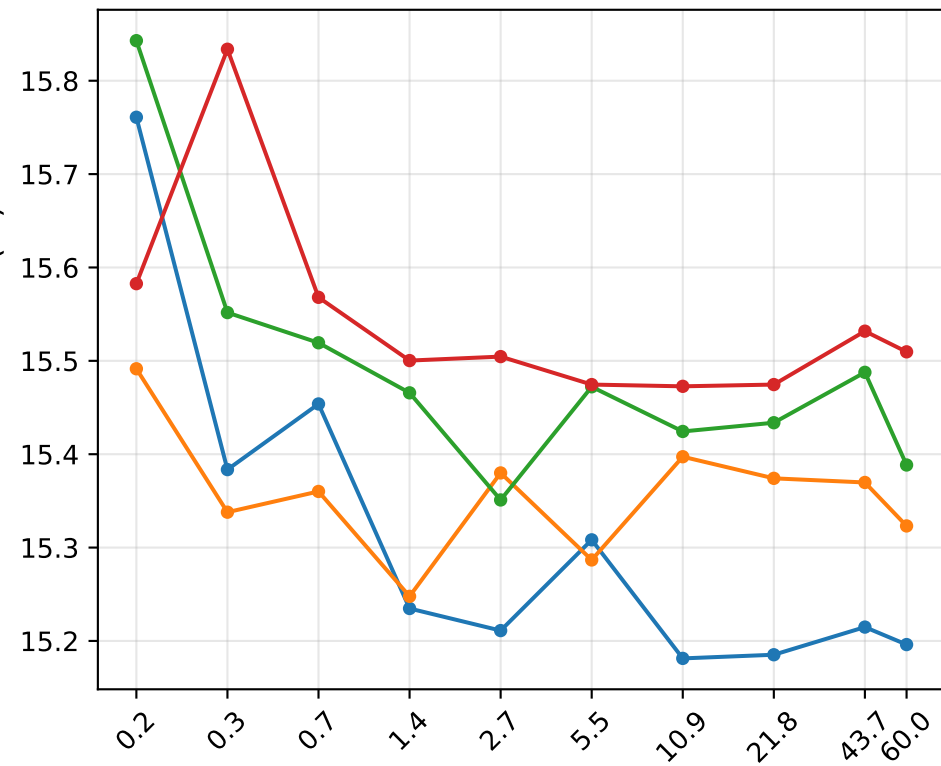
Rev16
