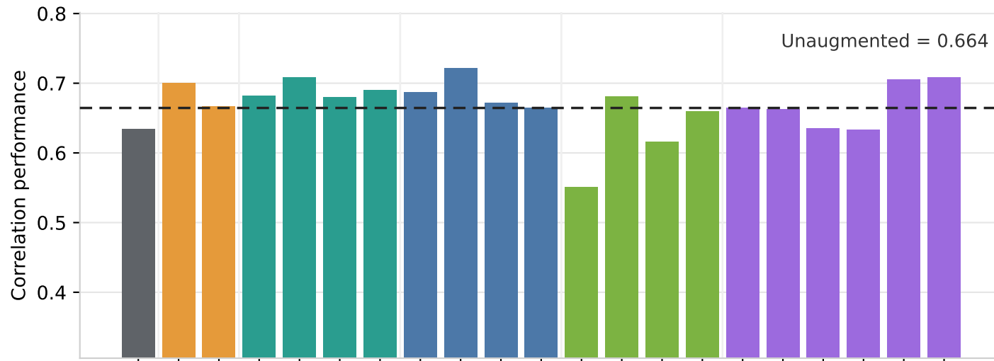
Claude Sonnet 4.6
