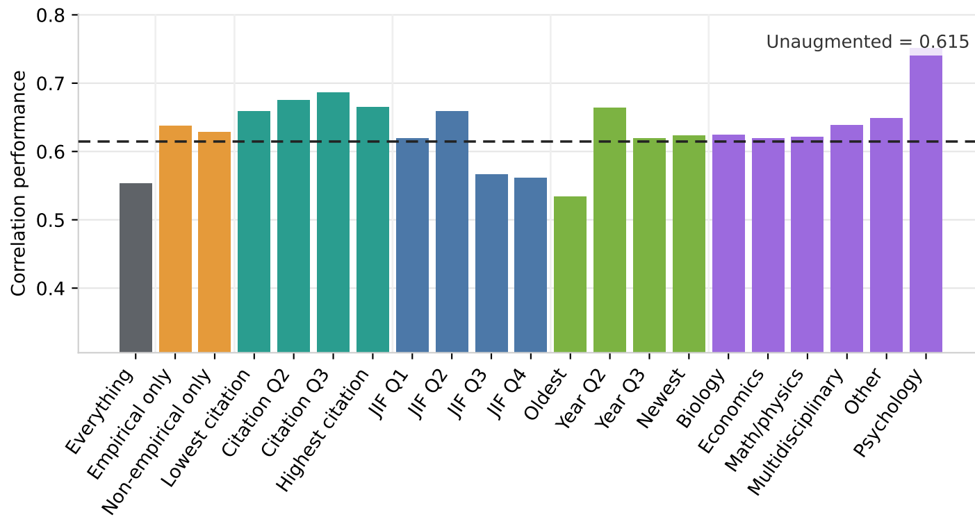
GPT-4.1
