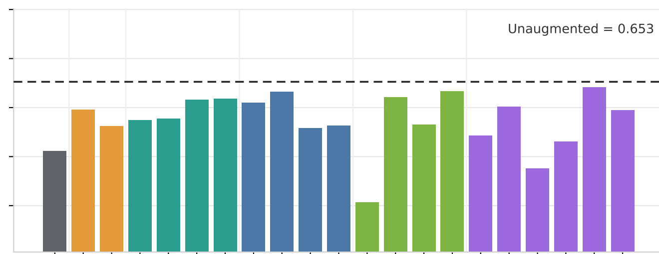
GPT-5.1
