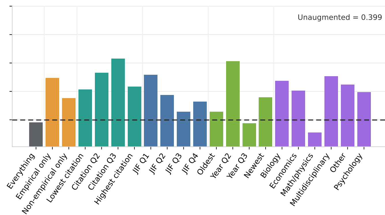
Gemini 2.5 Pro
