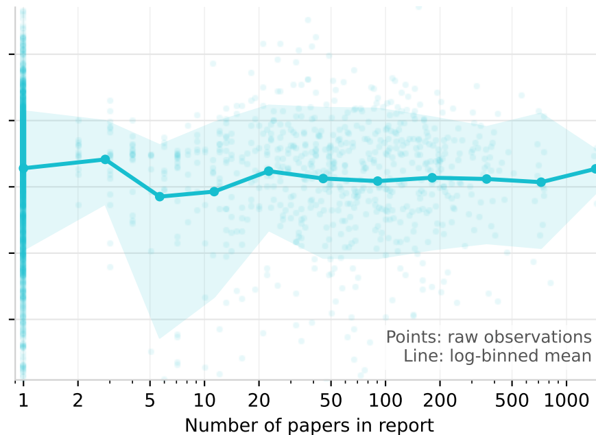
Gemini 2.5 Pro
