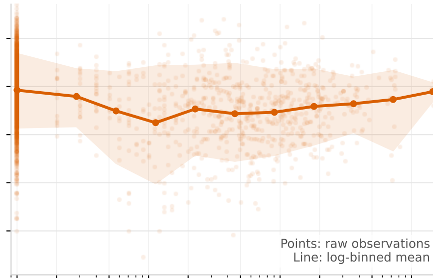
GPT-5.1
