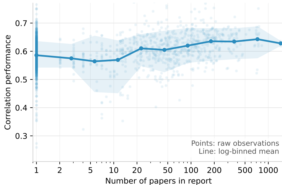
GPT-4.1
