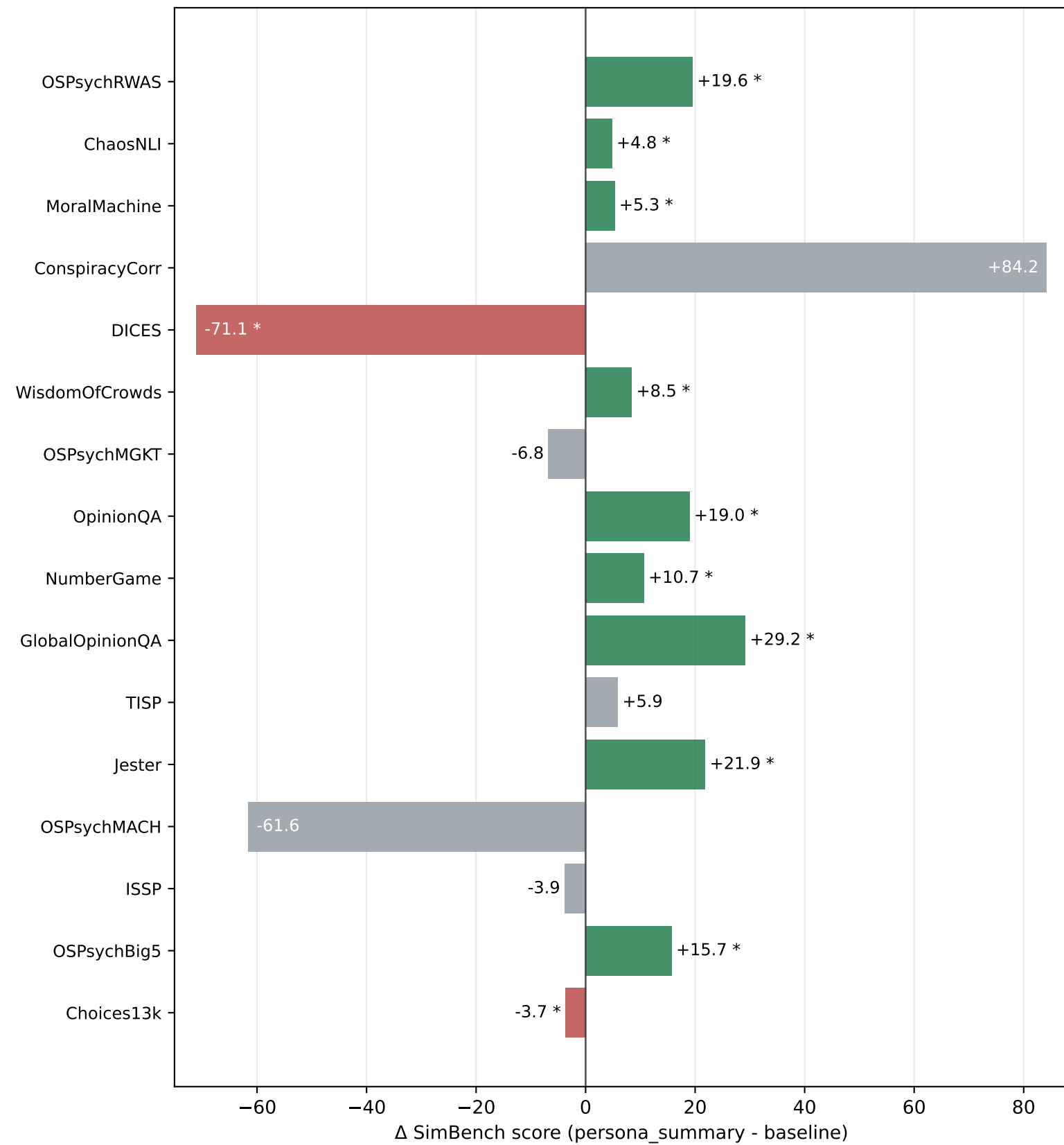
gpt-5-nano
