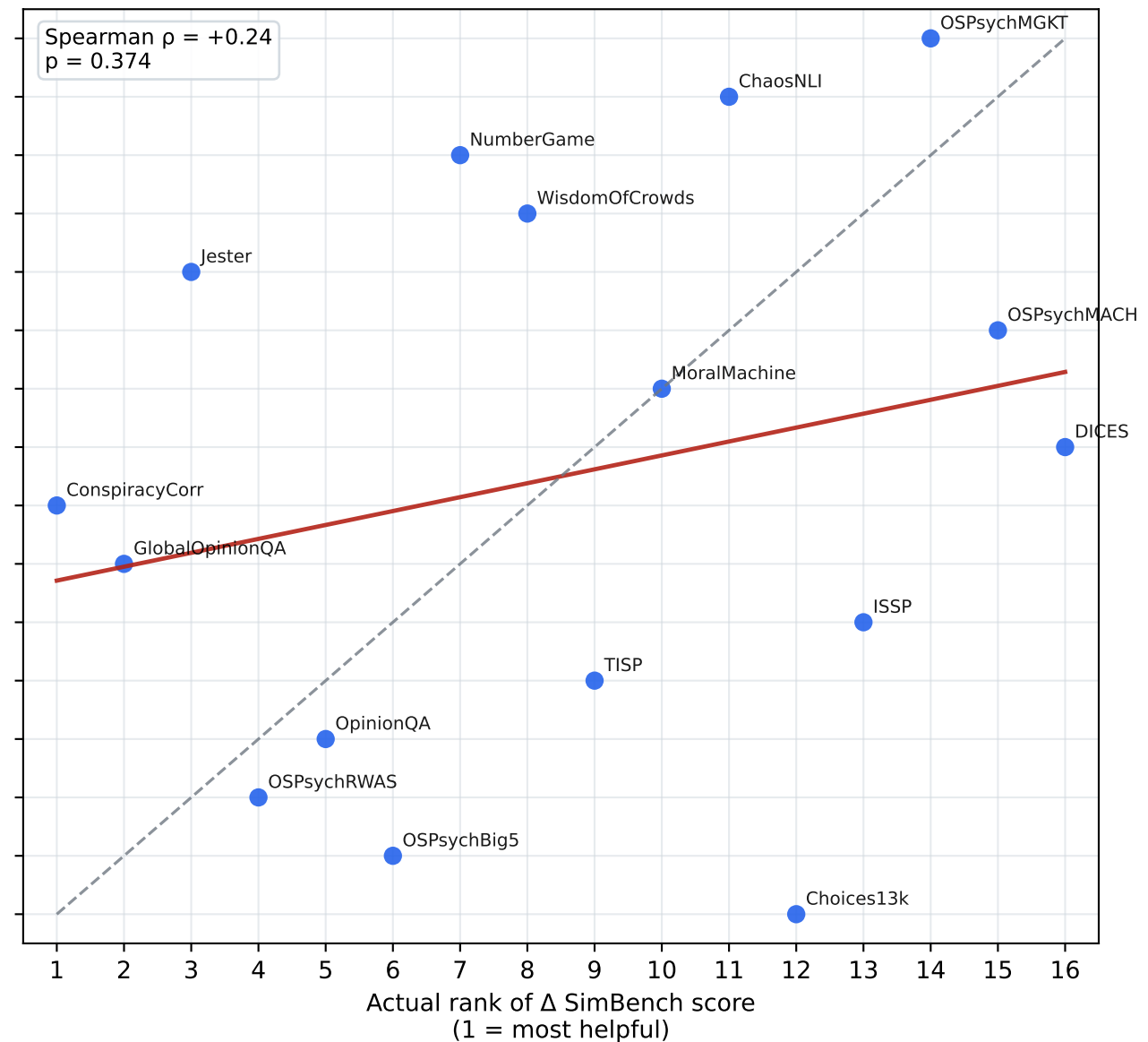
gpt-5-nano
