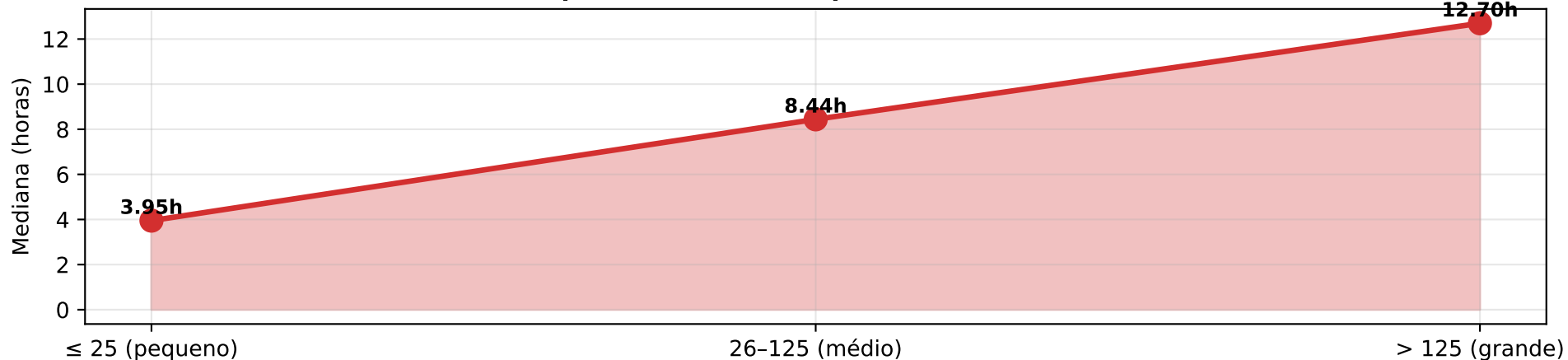
Tempo até Fechamento por Faixa de LOC (S4)
