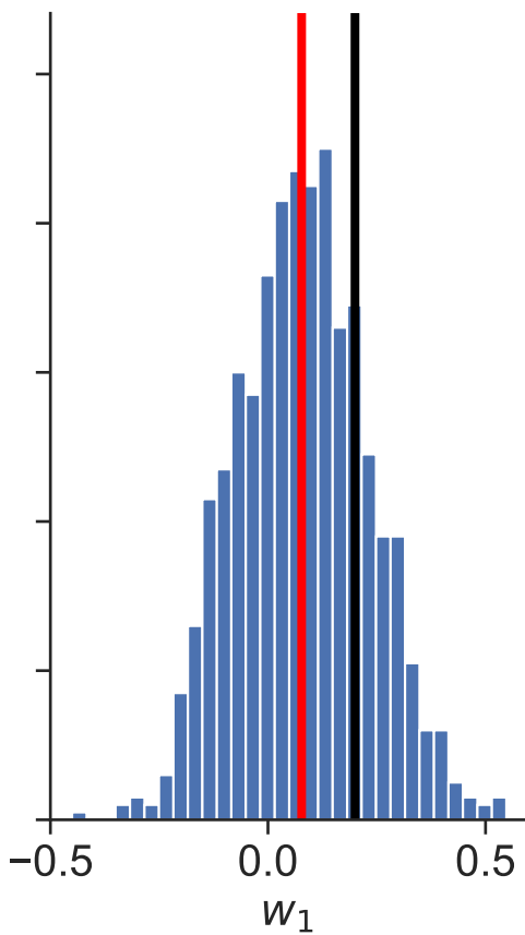
Posterior distributions Dataset 45
