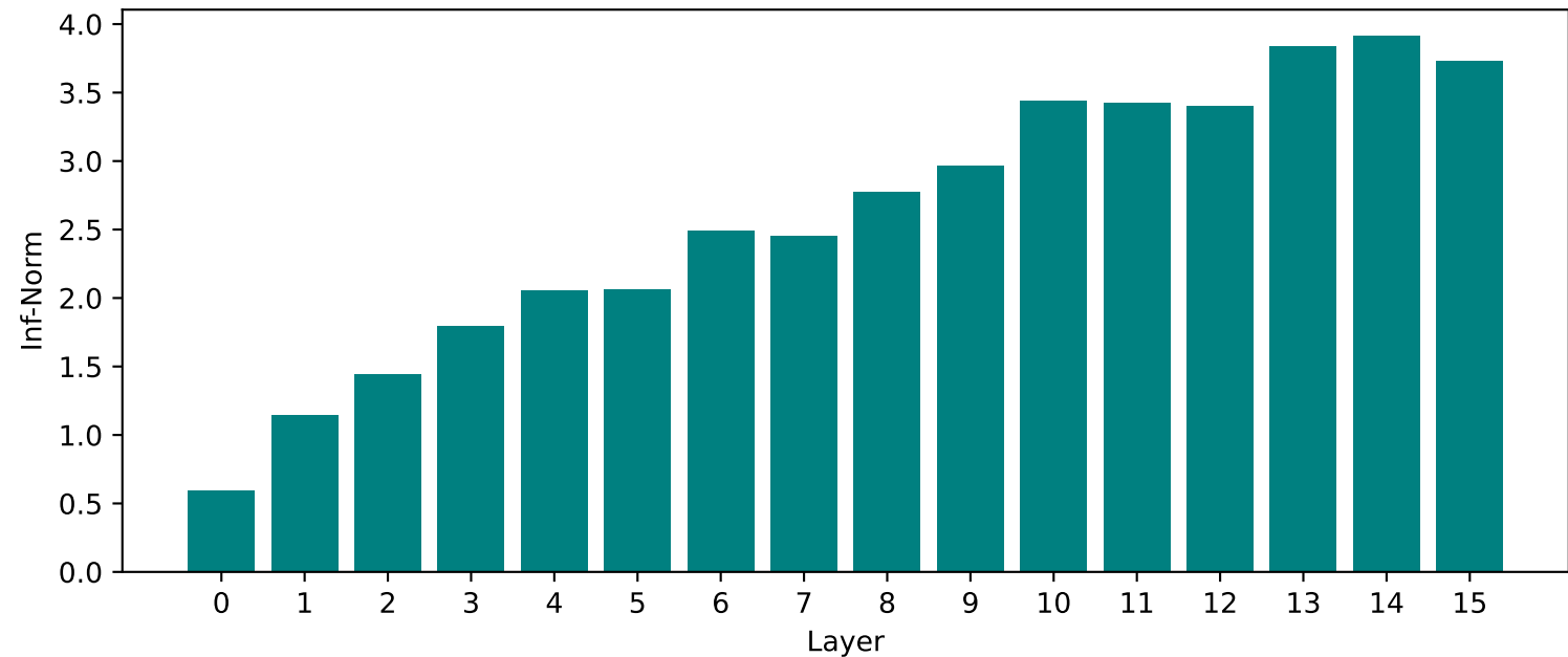
Hidden State Inf-Norm per Layer
