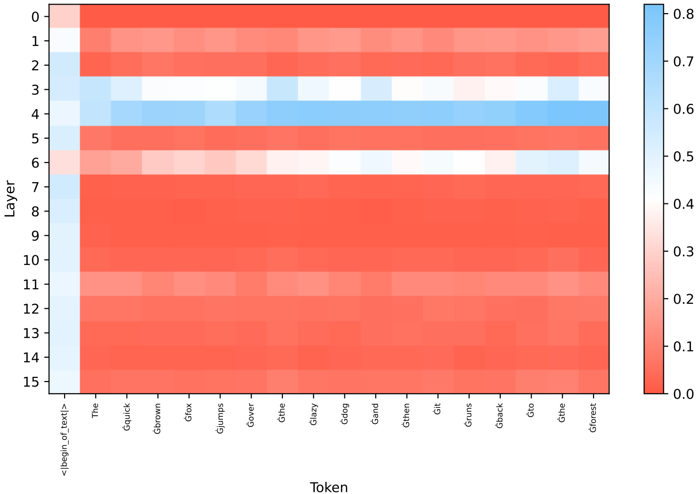
OASIS: Null Posterior per Token per Layer
