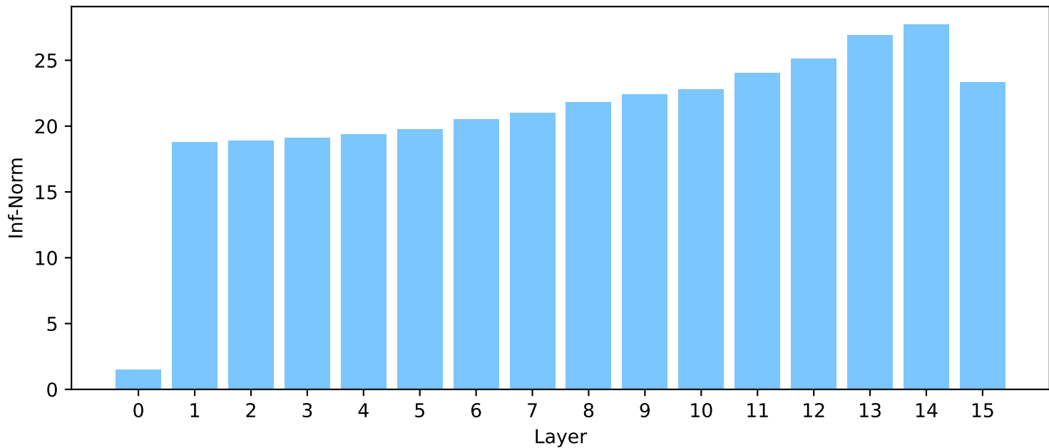
Hidden State Inf-Norm per Layer
