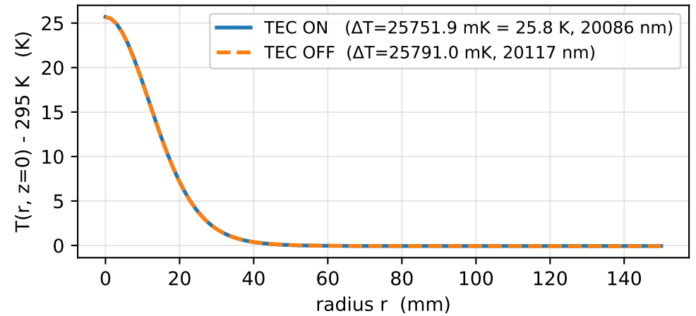
(d) STATIONARY case -- wafer-top profile (worst-case)
