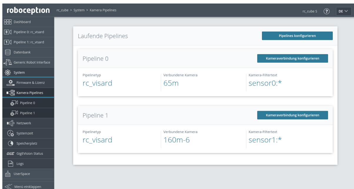
Abb. 5.1: Beispiel der Seite Kamera Pipelines auf einem rc_cube mit zwei laufenden Pipelines vom Typ rc_visard
