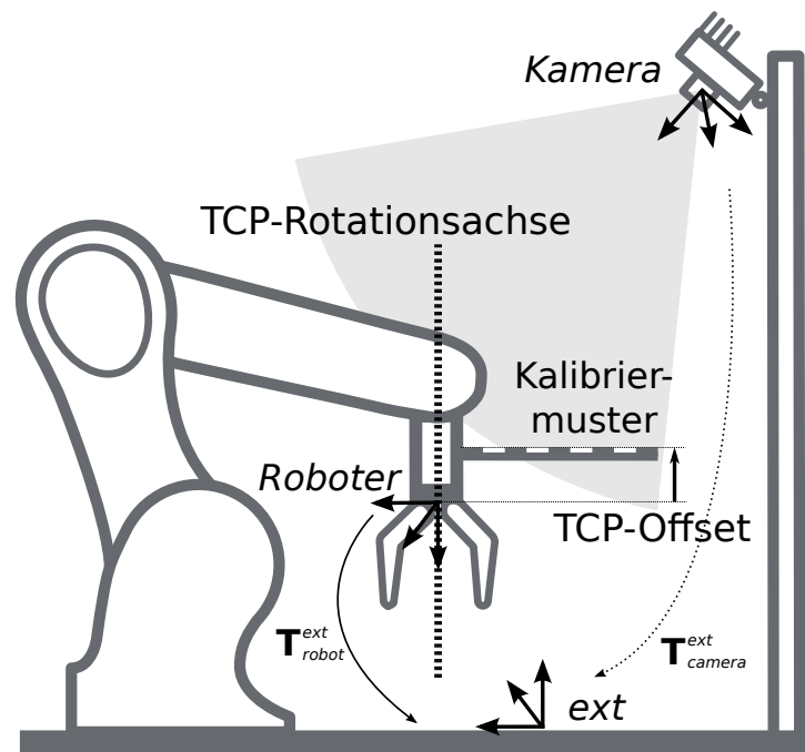
Abb. 6.19: Im Fall eines 4DOF-Roboters müssen die TCP-Rotationsachse und der Offset vom TCP zur sichtbaren Oberfläche des Kalibrieramusters entlang der TCP-Rotationsachse angegeben werden. Im dargestellten Fall ist der Offset negativ.
