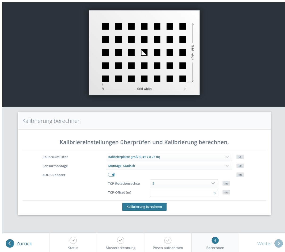
Abb. 6.24: Setzen der Parameter und Berechnen der Hand-Auge-Kalibrierung in der Web GUI des rc_cube
