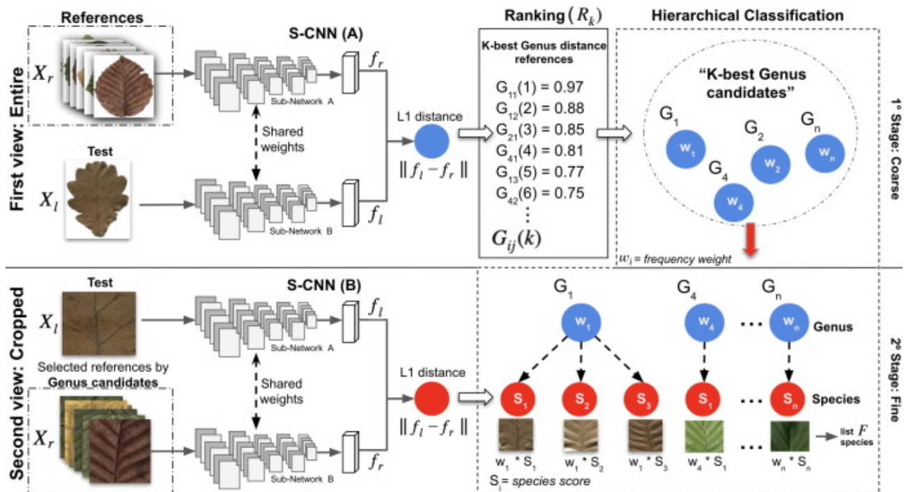
Рисунок 3.8 – Иерархическая классификация с использованием SCNN
