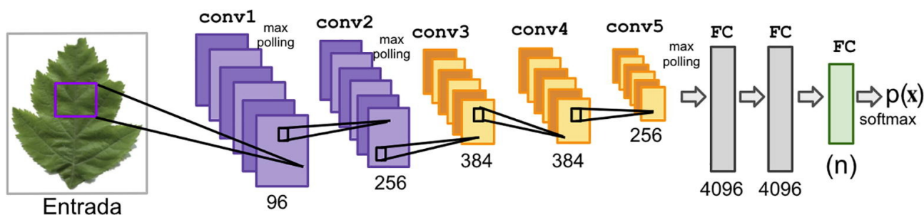
Рисунок 3.4 – Архитектура AlexNet
