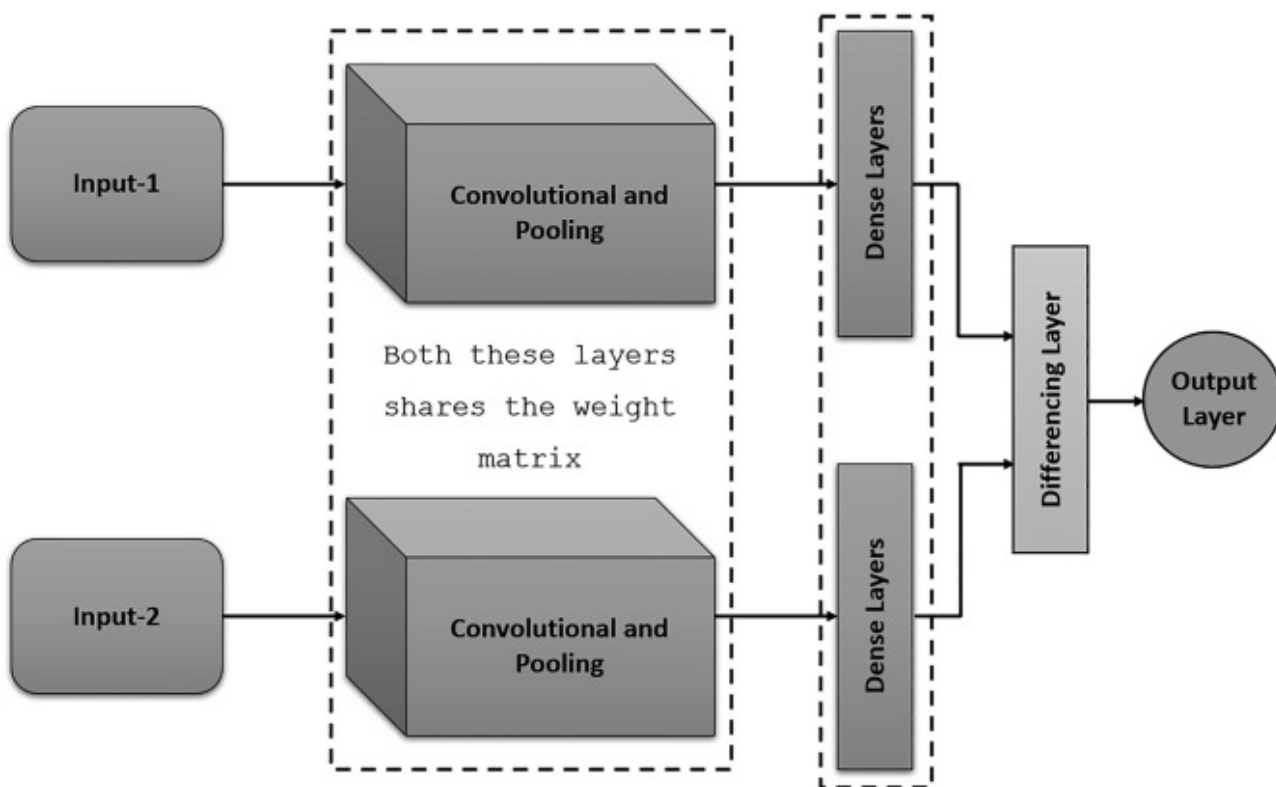
Рисунок 3.7 – Архитектура SCNN
