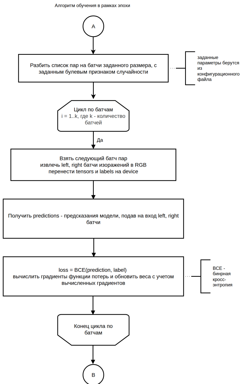
Рисунок 2.6 – Схема алгоритма обучения сиамских моделей, часть 6
