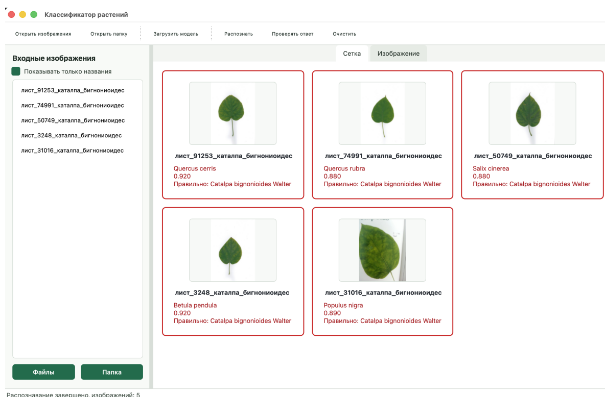
Рисунок 3.4 – Отображение результатов классификации в сетке
