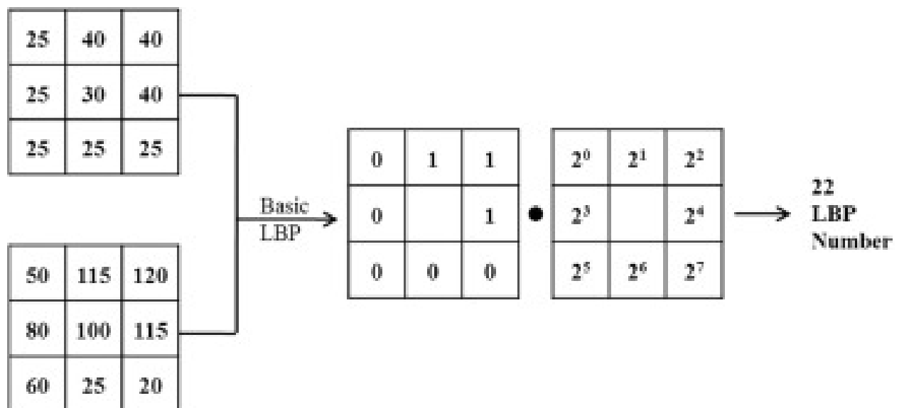
Рисунок 1.5 – Пример вычисления LBP-кода пикселя
