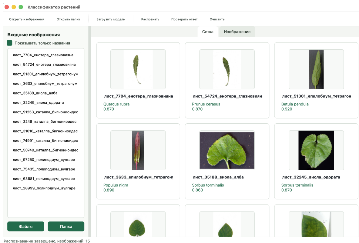
Рисунок 3.1 – Представление результатов классификации в виде сетки
