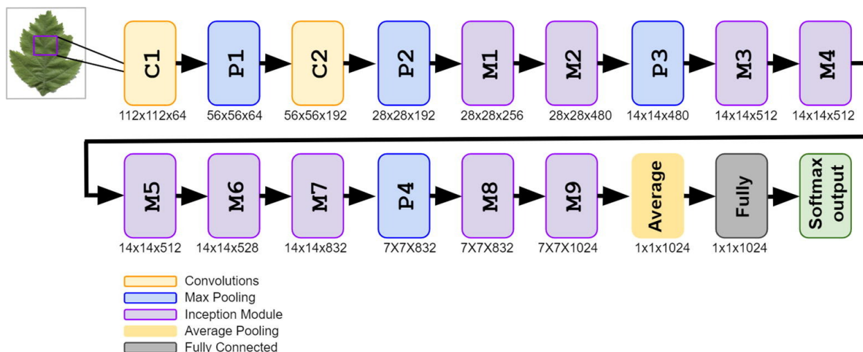
Рисунок 1.8 – Архитектура GoogLeNet
