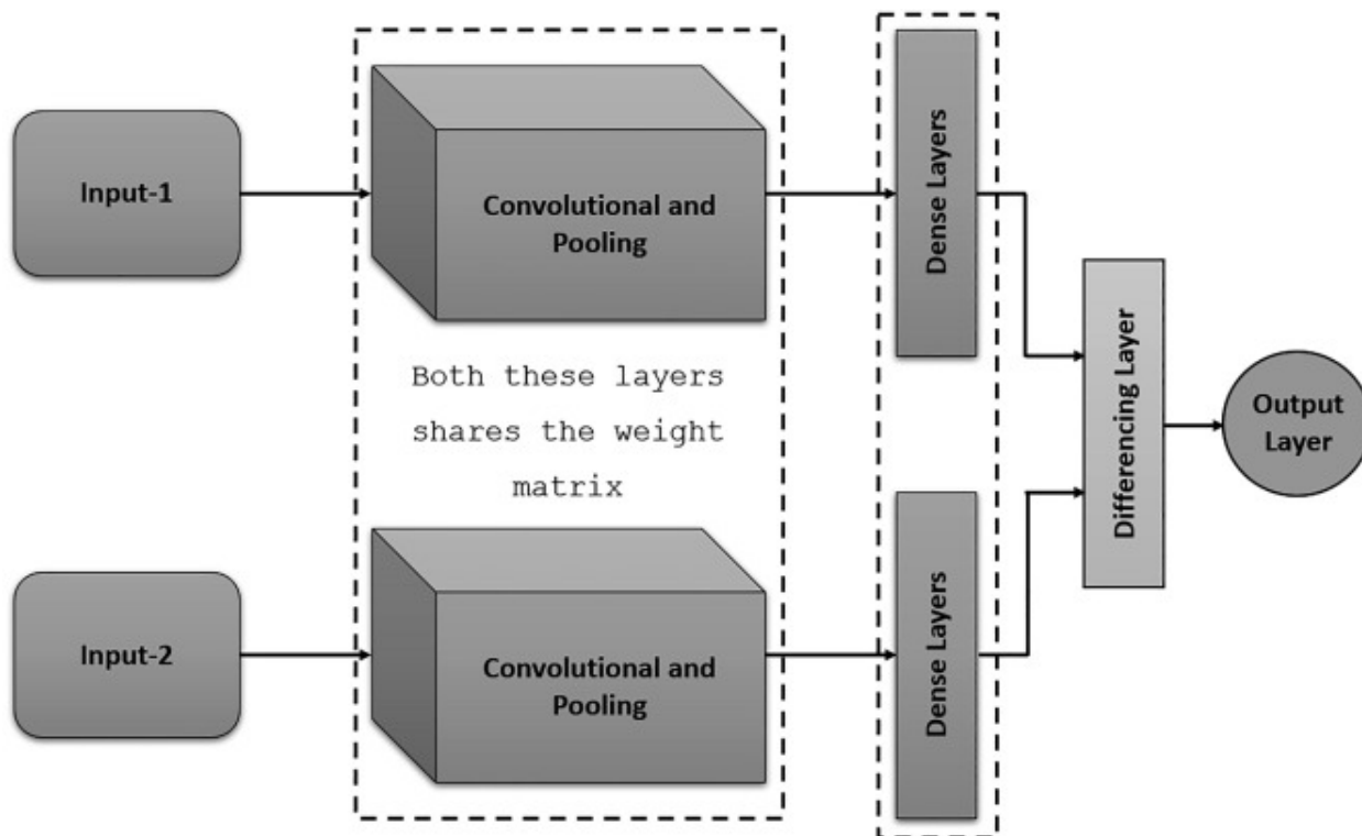
Рисунок 1.10 – Архитектура SCNN
