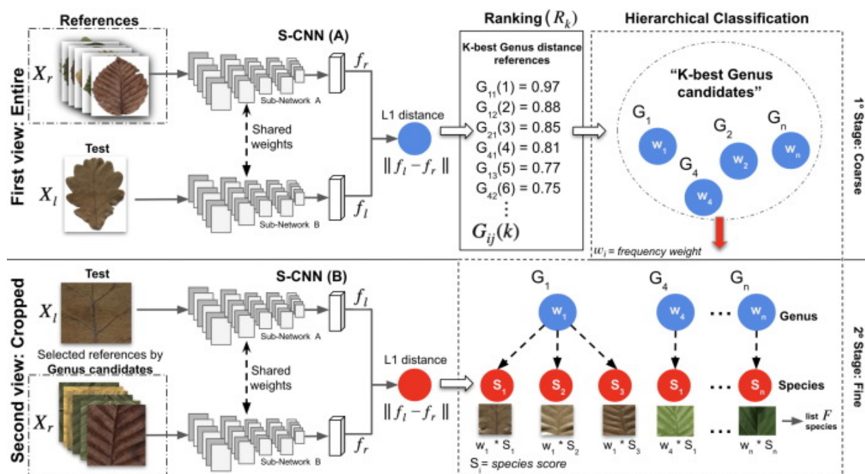
Рисунок 1.11 – Иерархическая классификация с использованием SCNN
