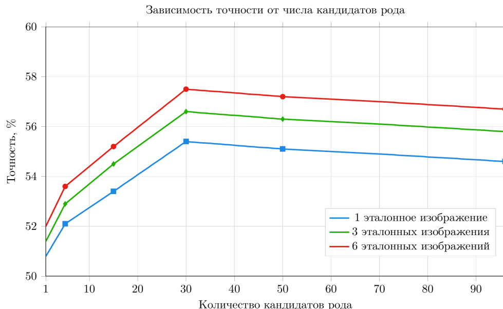
Рисунок 4.1 – Зависимость точности от числа кандидатов рода при различном числе эталонных изображений
