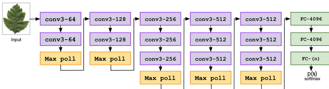
Рисунок 1.9 – Архитектура VGGNet
