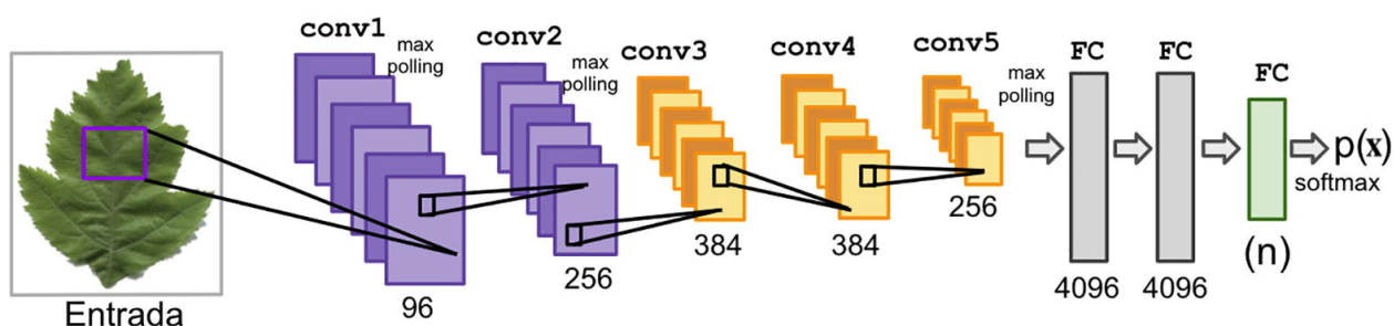
Рисунок 1.7 – Архитектура AlexNet
