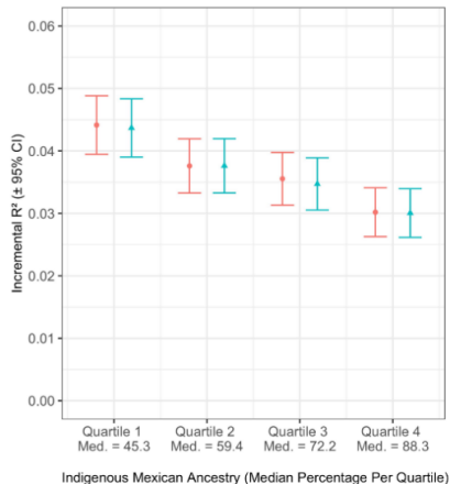
Figura 5: Decaimiento de precisión de PGS en MCPS. Los PGS derivan de UKB y decaen con el porcentaje de ancestría indígena mexicana (Ziyatdinov et al. 2023, Nature ).
