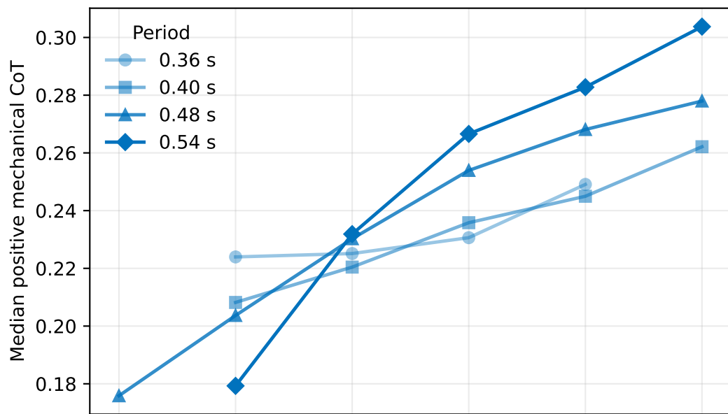
Trot
