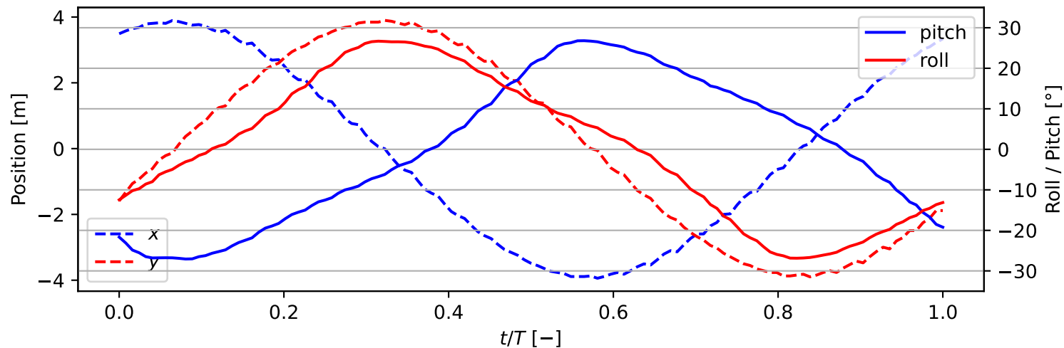
Circular Trajectory r = 3m , v = 3m/s
