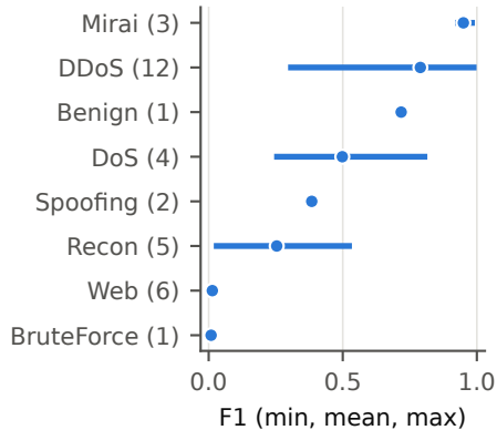
CICIoT2023
