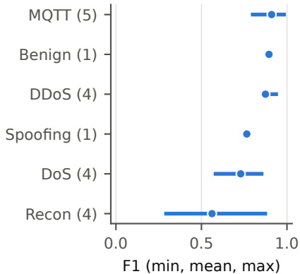
CICIoMT2024
