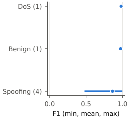
CICIoV2024
