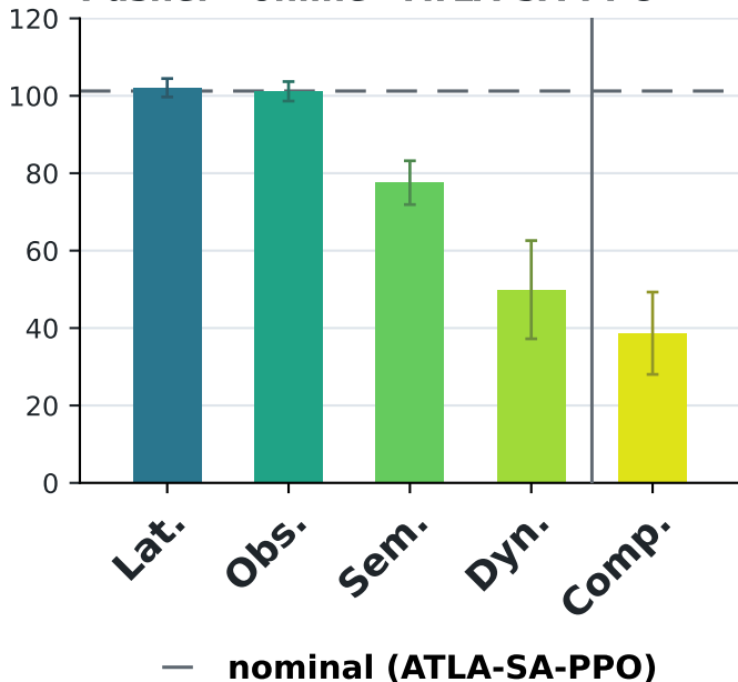
Pusher · online · ATLA-SA-PPO
