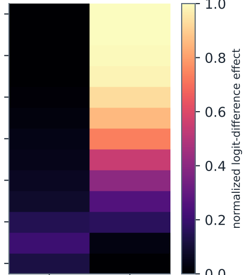
XGLM-564M
