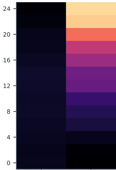
Qwen3-0.6B
