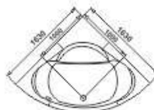
ZEM NX Size : 1630 x 1630 x 2200 mm
