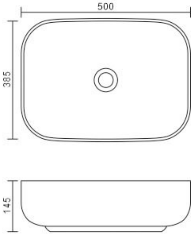
Size : 500 x 385 x 145 mm
