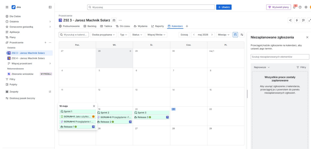
Rysunek 13: Widok zakładki kalendarza prezentujący ukończone epiki, historyjki oraz poszczególne sprinty
