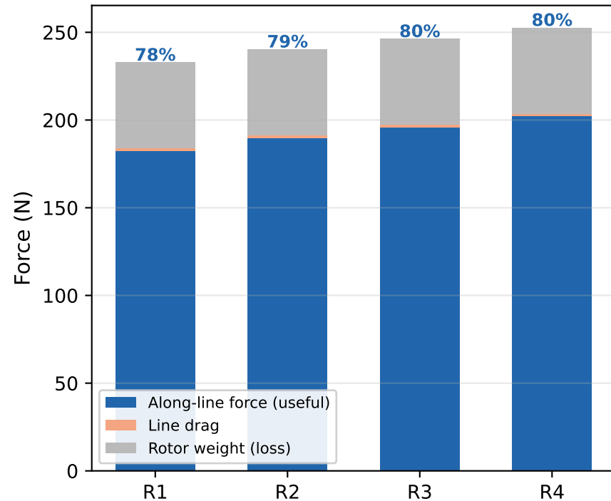
Force Budget per Rotor R=3.0m, N=4, 8 m/s
