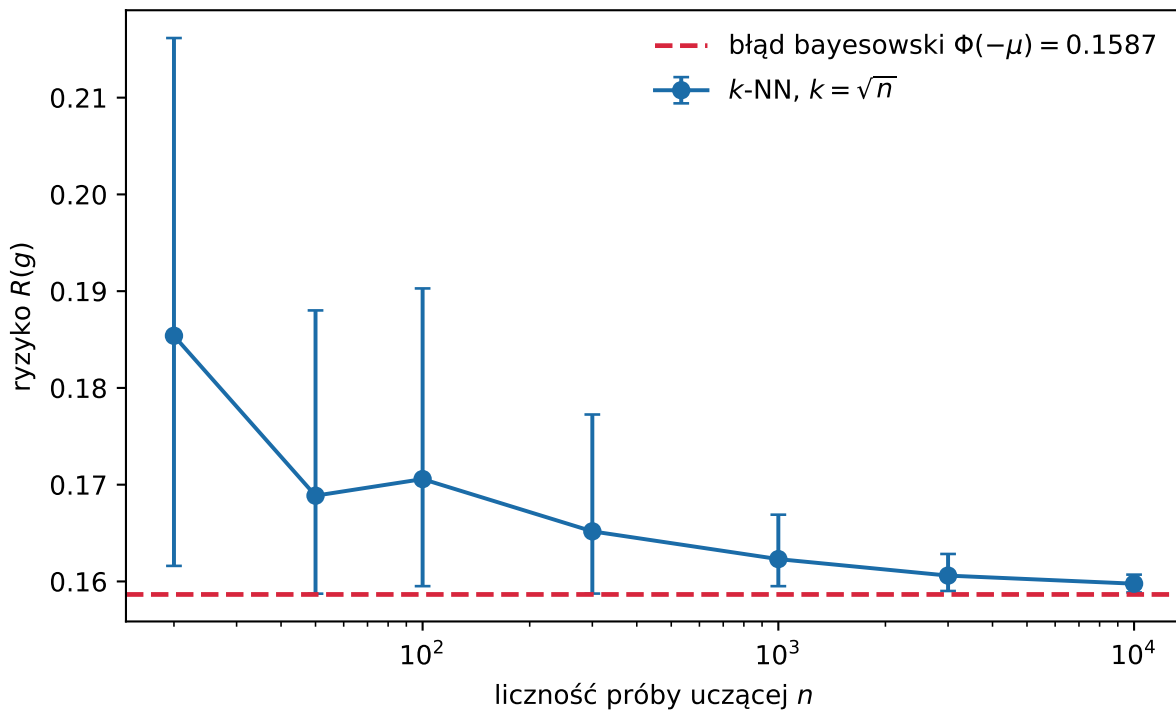
Rysunek 2.2.: Ryzyko klasyfikatora k -NN w zależności od liczności próby uczącej, dla dwóch klas \mathcal{N}(\pm 1, 1) . Punkty to średnie z 25 niezależnych prób uczących, wąsy – kwantyle rzędu 0,1 i 0,9. Błąd bayesowski \Phi(-1) \approx 0,1587 wyznacza poziom, poniżej którego nie schodzi żaden klasyfikator, niezależnie od liczby obserwacji.
