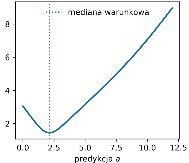
strata absolutna |y - a|
