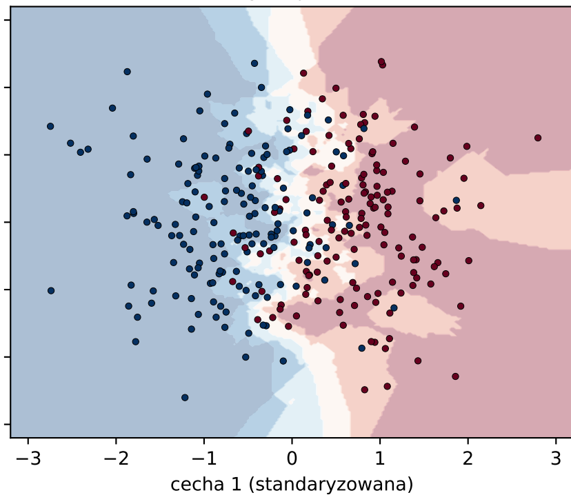
ze standaryzacją: błąd 0.167
