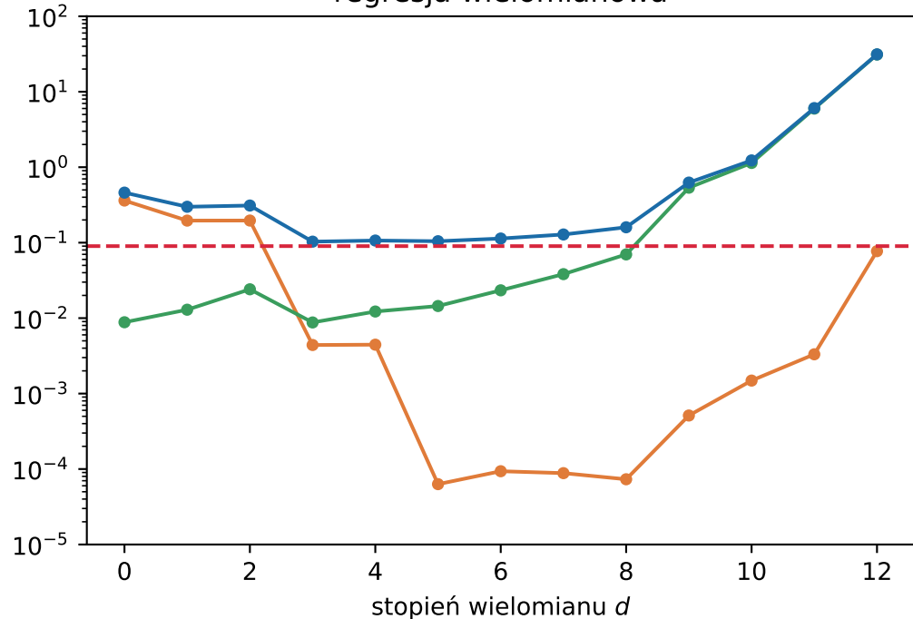
regresja wielomianowa
