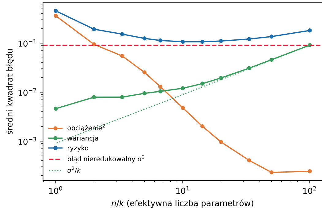
k -NN
