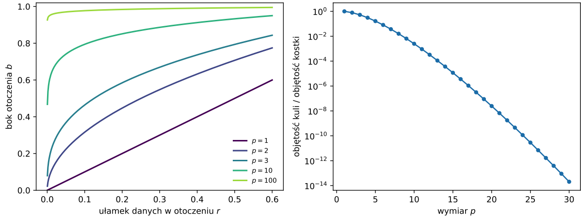
Rysunek 3.7.: Geometria wysokich wymiarów. Po lewej: bok kostki-otoczenia, które obejmuje ułamek r danych jednostajnych w [0, 1]^p , według wzoru b = r^{1/p} . Po prawej: ułamek objętości kostki zajmowany przez kulę wpisaną (oś pionowa w skali logarytmicznej).
