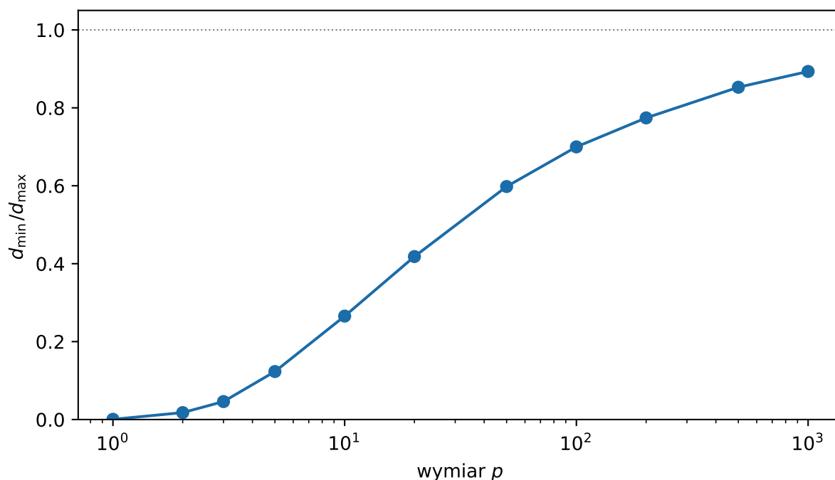
Rysunek 3.8.: Koncentracja odległości. Dla n = 1000 punktów jednostajnych w [0, 1]^p i losowego punktu zapytania pokazano iloraz odległości do najbliższego i najdalszego punktu (średnia z 50 punktów zapytania). Gdy iloraz zbliża się do 1, najbliższy i najdalszy sąsiad są od punktu niemal tak samo odlegli.
