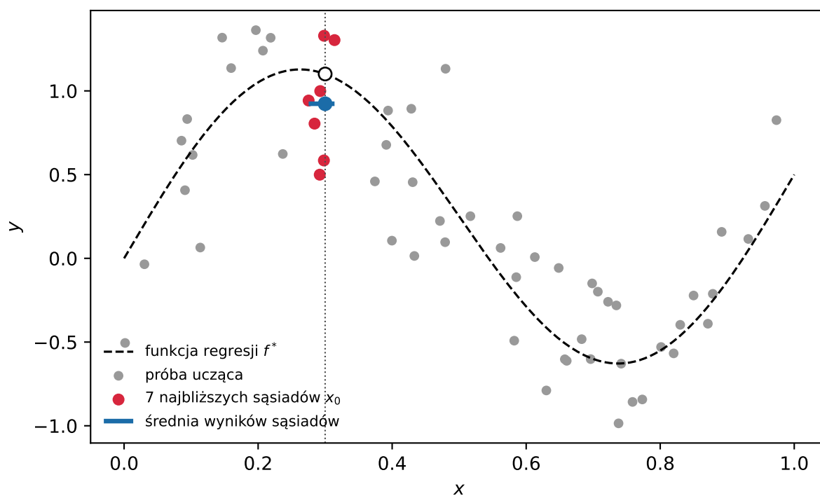
Rysunek 3.1.: Uśrednianie lokalne. Szare punkty to próba ucząca, przerywana krzywa – prawdziwa funkcja regresji f^* . Aby przewidzieć wynik w punkcie x_0 , wybieramy k = 7 obserwacji o cechach najbliższych x_0 (zaznaczone na czerwono) i uśredniamy ich wyniki. Pozioma kreska pokazuje tę średnią na przedziale zajmowanym przez sąsiadów.
