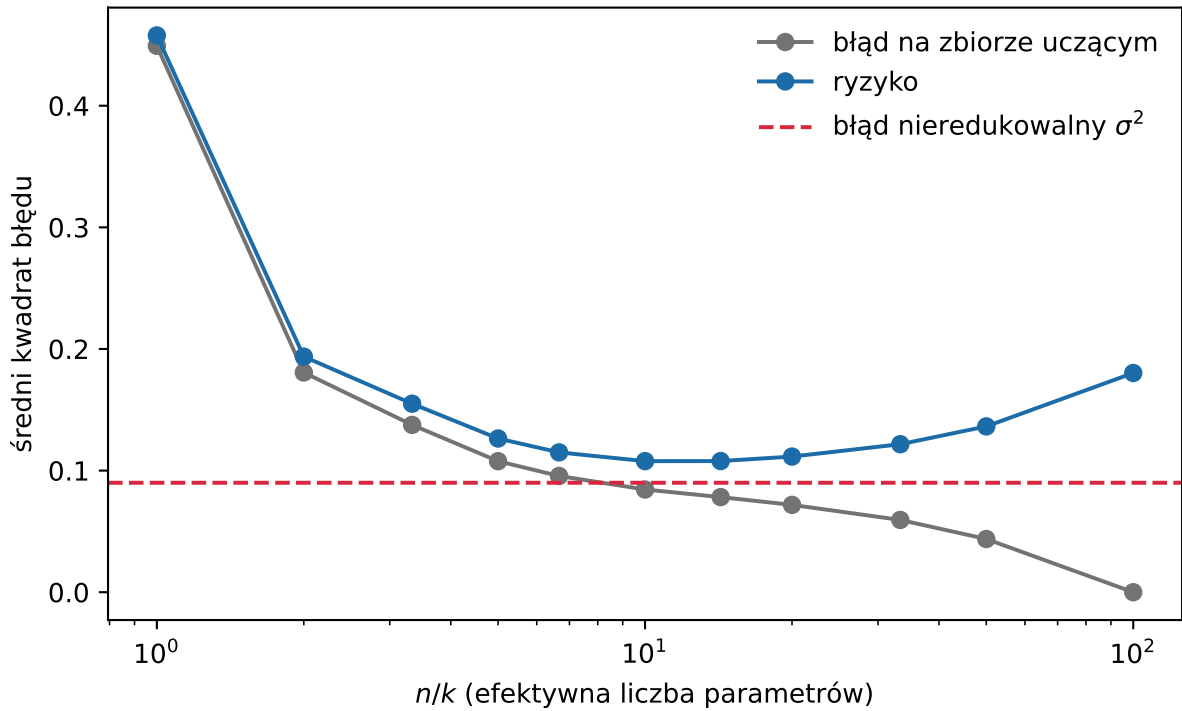
Rysunek 3.5.: Błąd na zbiorze uczącym i ryzyko regresji k -NN w zależności od n/k ( n = 100 ). Ryzyko policzono dokładnie, całkując po znanym rozkładzie. Punkty to średnie z 50 niezależnych prób uczących. Przerywana linia to błąd nieredukowalny \sigma^2 .
