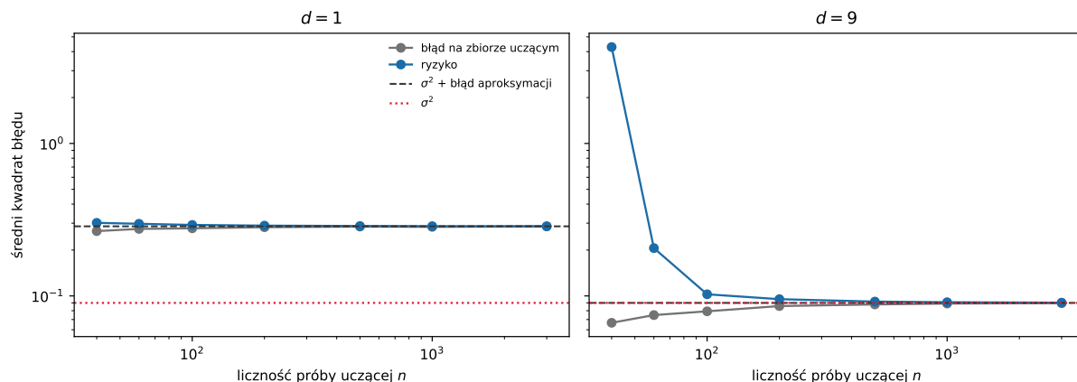
Rysunek 4.4.: Krzywe uczenia regresji wielomianowej stopnia d = 1 (po lewej) i d = 9 (po prawej): błąd na zbiorze uczącym i ryzyko w zależności od liczności próby n . Punkty to średnie z 300 prób uczących. Linia przerywana: granica ryzyka przy n \rightarrow \infty , równa sumie błędu nieredukowalnego i błędu aproksymacji. Linia kropkowana: błąd nieredukowalny \sigma^2 . Obie osie w skali logarytmicznej.
