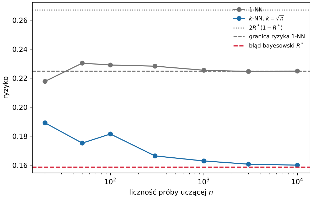
Rysunek 3.6.: Ryzyko reguły 1-NN i reguły k -NN z k = \sqrt{n} w zależności od liczności próby, dla dwóch klas \mathcal{N}(\pm 1, 1) . Ryzyko policzono dokładnie, całkując po znanym rozkładzie; punkty to średnie z 25 prób uczących. Linie poziome: błąd bayesowski R^* , granica ryzyka 1-NN z twierdzenia Covera–Harta i jej ograniczenie górne 2R^*(1 - R^*) .
