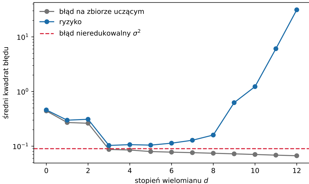
Rysunek 4.1.: Błąd na zbiorze uczącym i ryzyko regresji wielomianowej w zależności od stopnia wielomianu d ( n = 50 ). Ryzyko policzono dokładnie, całkując po znanym rozkładzie; punkty to średnie z 1000 niezależnych prób uczących. Oś pionowa w skali logarytmicznej. Przerywana linia to błąd nieredukowalny \sigma^2 .
