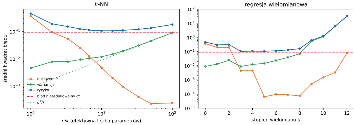
Rysunek 4.3.: Rozkład ryzyka na obciążenie do kwadratu, wariancję i błąd nieredukowalny. Po lewej: regresja k -NN w zależności od n/k ( n = 100, 500 prób uczących); kropkowana linia to wariancja \sigma^2/k z ustalonego układu (4.6). Po prawej: regresja wielomianowa w zależności od stopnia d ( n = 50, 1000 prób uczących, te same co na rysunku 4.1). Ryzyko jest sumą trzech składników. Oś pionowa w skali logarytmicznej.
