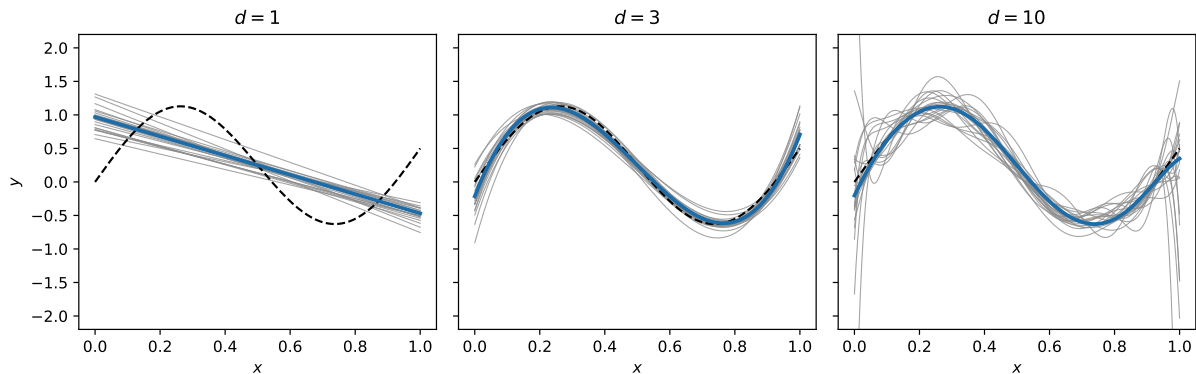
Rysunek 4.2.: Wielomiany stopni d = 1, 3, 10 dopasowane do 20 niezależnych prób uczących liczących n = 50 (cienkie linie). Gruba niebieska linia to predyktor przeciętny \bar{f} , oszacowany z 1000 prób, przerywana – funkcja regresji f^* .
