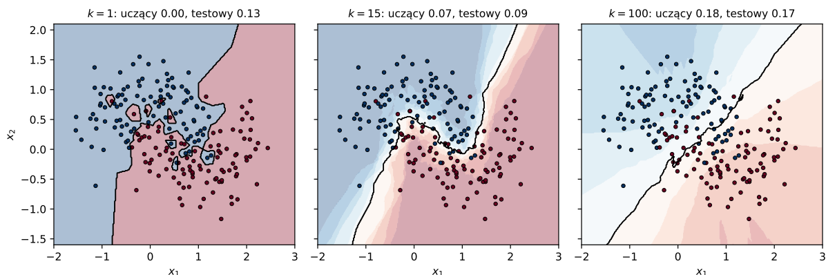
Rysunek 3.3.: Klasyfikator k -NN dla k = 1, 15, 100 na zbiorze dwóch półksiężyców ( n = 200 , szum 0,30 ). Tło pokazuje oszacowanie \hat{\eta}(\mathbf{x}) , czarna linia – granicę decyzyjną \hat{\eta}(\mathbf{x}) = 1/2 . W tytułach podano błąd na zbiorze uczącym i na dużym zbiorze testowym z tego samego rozkładu.
