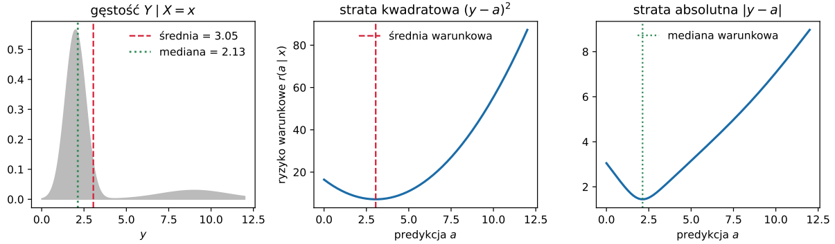
Rysunek 2.1.: Rozkład warunkowy Y | \mathbf{X} = \mathbf{x} i ryzyko warunkowe r(a | \mathbf{x}) jako funkcja predykcji a . Po lewej: gęstość mieszaniny 0,85 \mathcal{N}(2, 0,6^2) + 0,15 \mathcal{N}(9, 2^2) z zaznaczoną średnią i medianą. W środku: ryzyko przy stracie kwadratowej, minimalizowane przez średnią warunkową. Po prawej: ryzyko przy stracie absolutnej, minimalizowane przez medianę warunkową. Oba ryzyka policzono dokładnie ze wzorów dla rozkładu normalnego.
