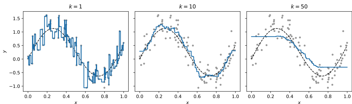
Rysunek 3.4.: Regresja k -NN dla k = 1, 10, 50 na tej samej próbie ( n = 100 ). Przerywana krzywa to funkcja regresji f^* , niebieska – predyktor \hat{f} .
