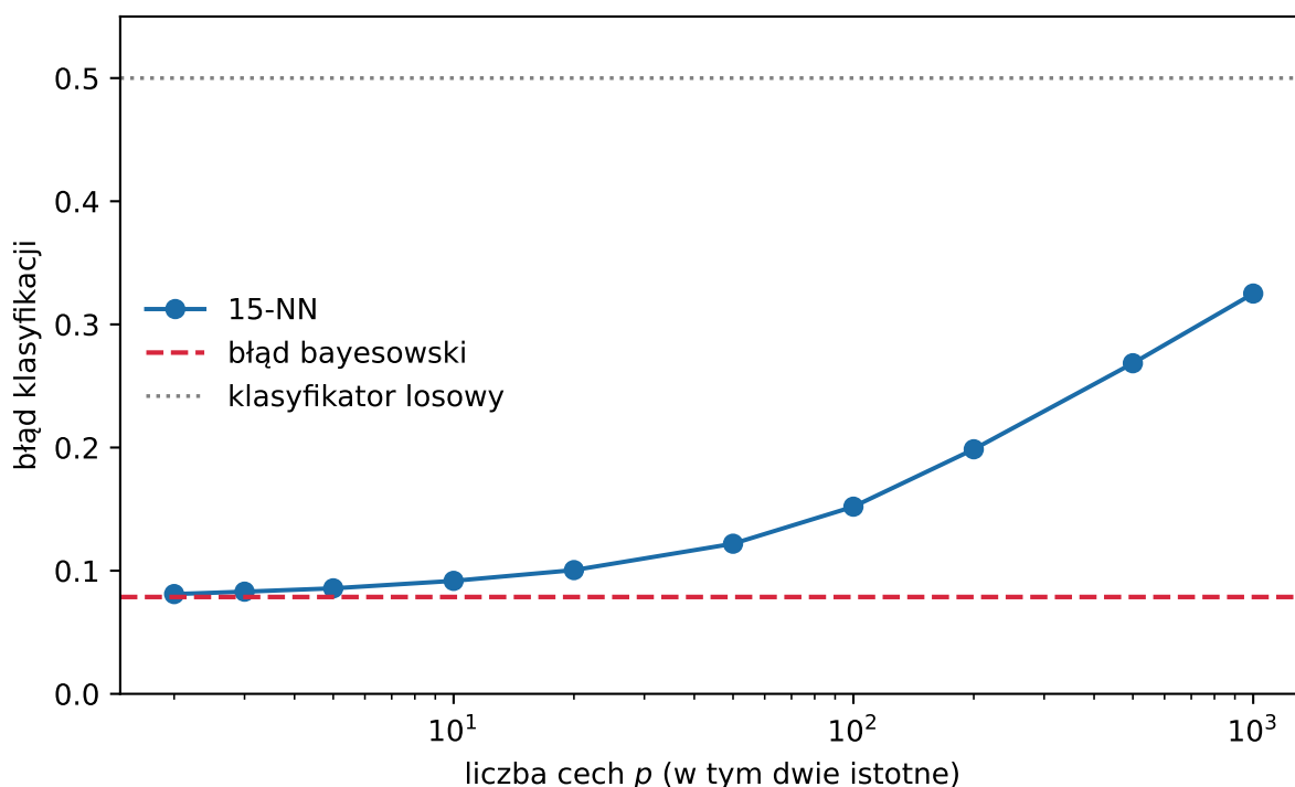
Rysunek 3.9.: Błąd klasyfikatora 15-NN w zależności od łącznej liczby cech p ( n = 500 , średnia z 5 prób uczących, błąd na zbiorze testowym liczności 10 000). Klasy różnią się tylko w dwóch pierwszych cechach, pozostałe p - 2 cech to szum. Linie poziome: błąd bayesowski, który nie zależy od cech nieistotnych, oraz błąd klasyfikatora losowego.
