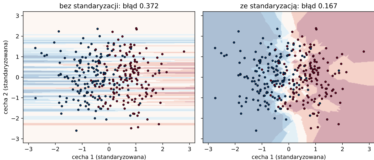
Rysunek 3.2.: Klasyfikator 5-NN bez standaryzacji (po lewej) i ze standaryzacją (po prawej), n = 300 . Klasę wyznacza tylko cecha 1. Cecha 2 jest szumem o odchyleniu standardowym 100, więc bez standaryzacji to ona decyduje o tym, kto jest czym sąsiadem. Oba panele narysowano w zmiennych standaryzowanych; tło pokazuje oszacowanie \hat{\eta}(\mathbf{x}) , a w tytule podano błąd na dużym zbiorze testowym.
