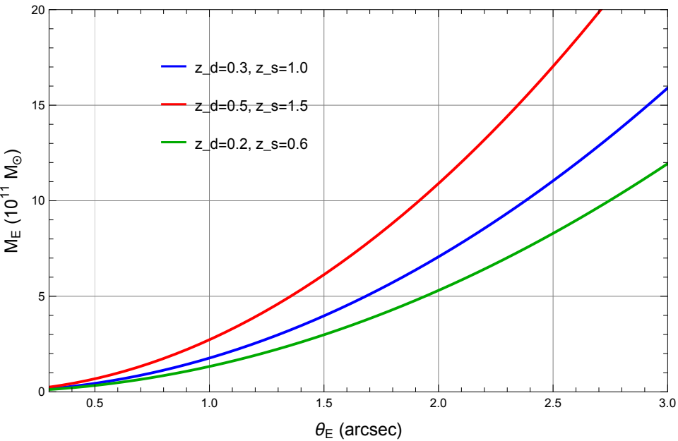
Einstein Mass vs Einstein Radius
