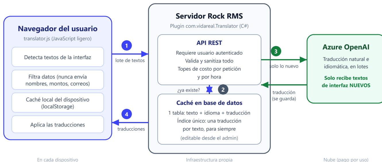
Fig. 1 — Arquitectura. El navegador nunca habla con Azure directamente; todo pasa por el servidor de Rock, que valida, aplica topes y cachea.
