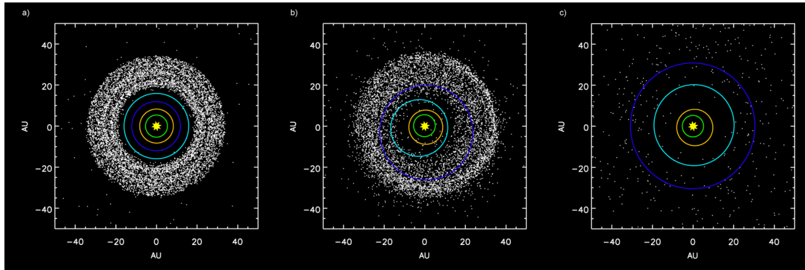
Simulación de los planetas exteriores y el cinturón de Kuiper, antes, durante y después de un salto orbital de Neptuno que produjo un bombardeo masivo en el resto de planetas
