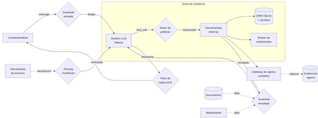
Figura 1: Diagrama de flujo de datos del agente y sus límites de confianza.
