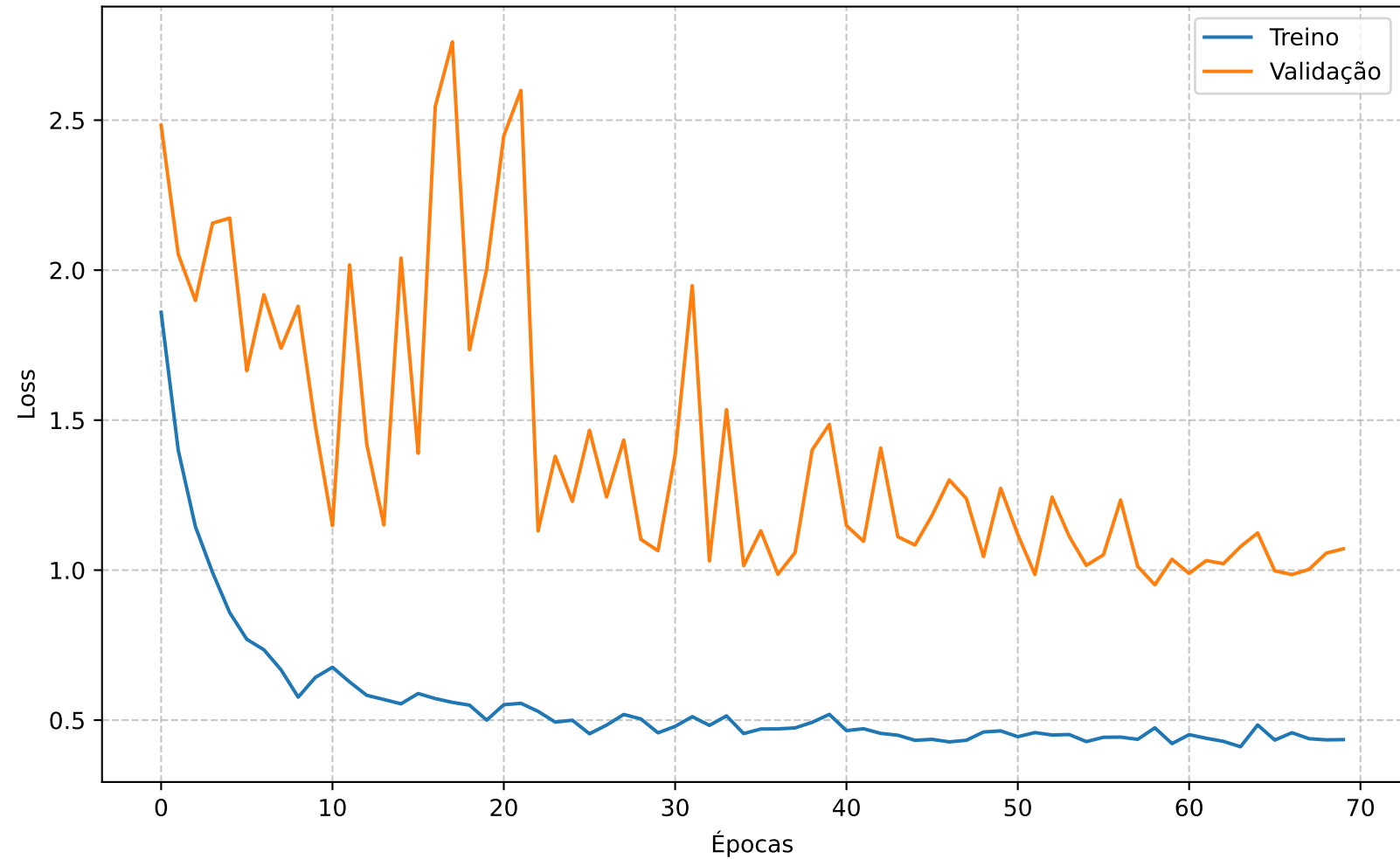
Curva de Aprendizado (Loss)
