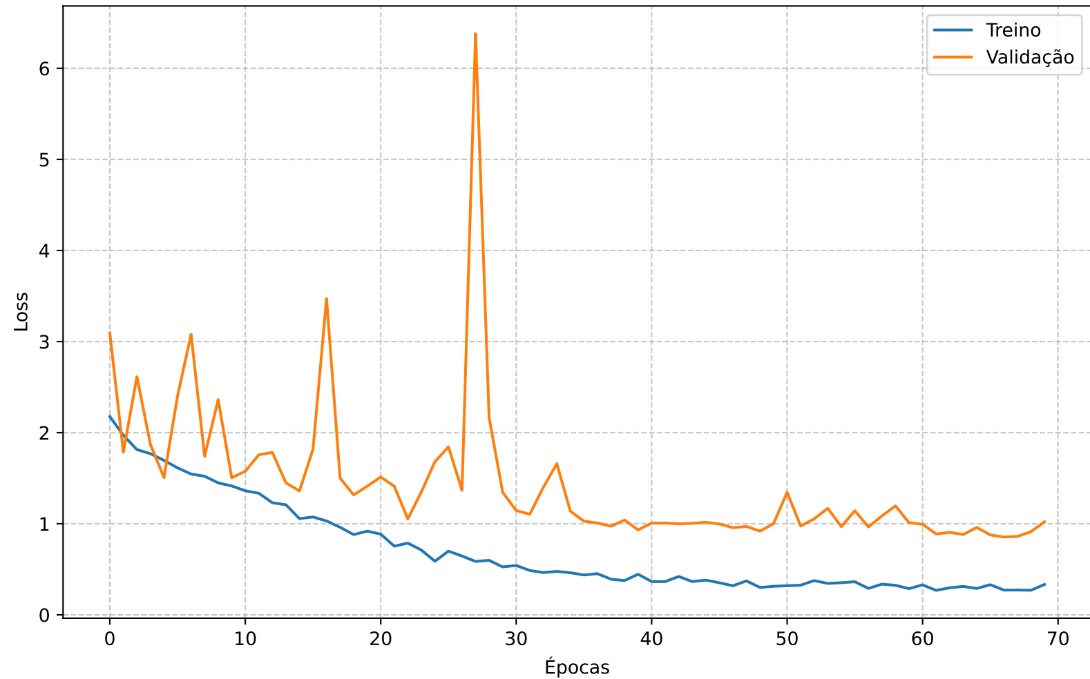
Curva de Aprendizagem (Loss)
