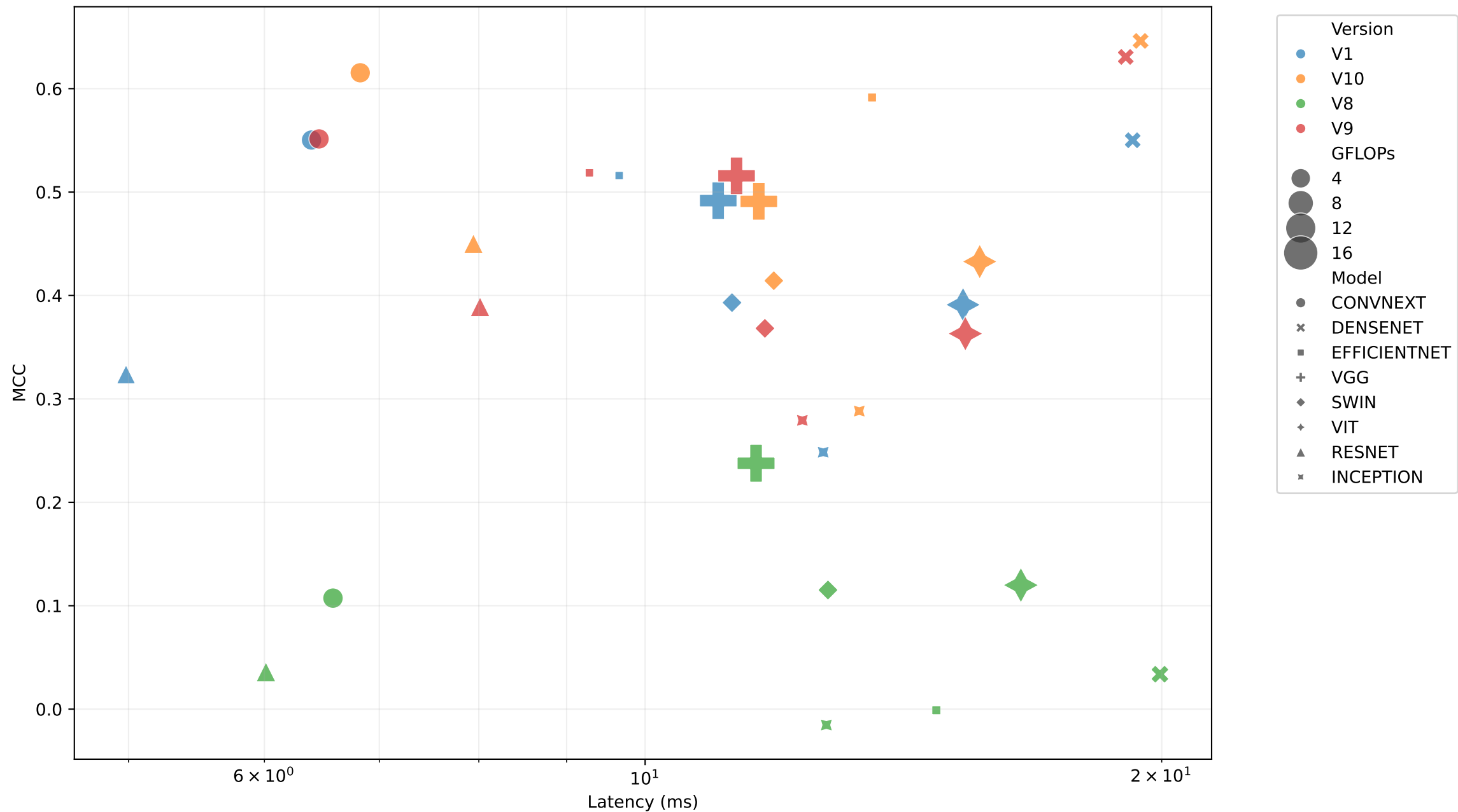
Trade-off Industrial: MCC vs Latência vs GFLOPs
