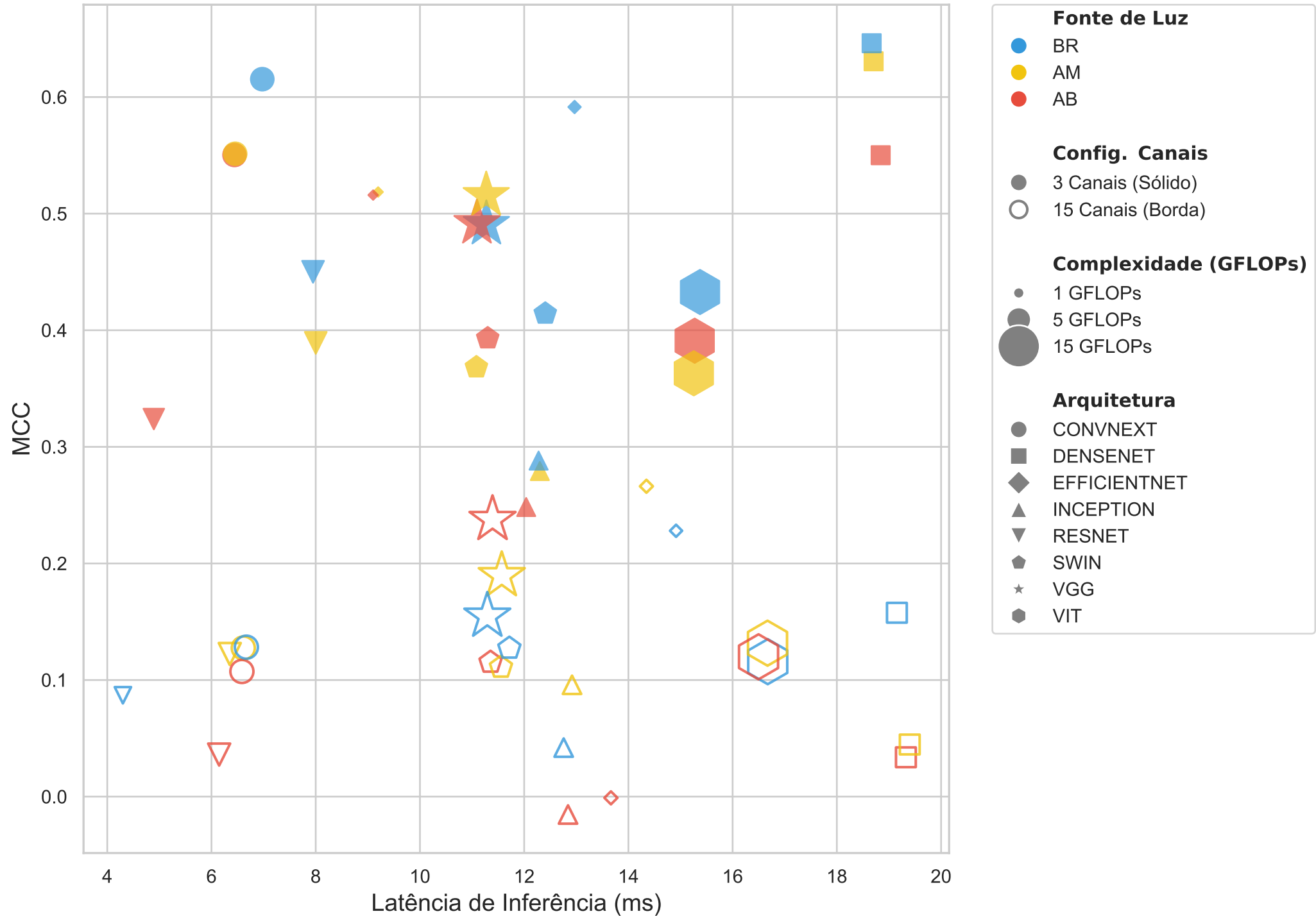
Trade-off Industrial: MCC vs. Latência vs. Complexidade
