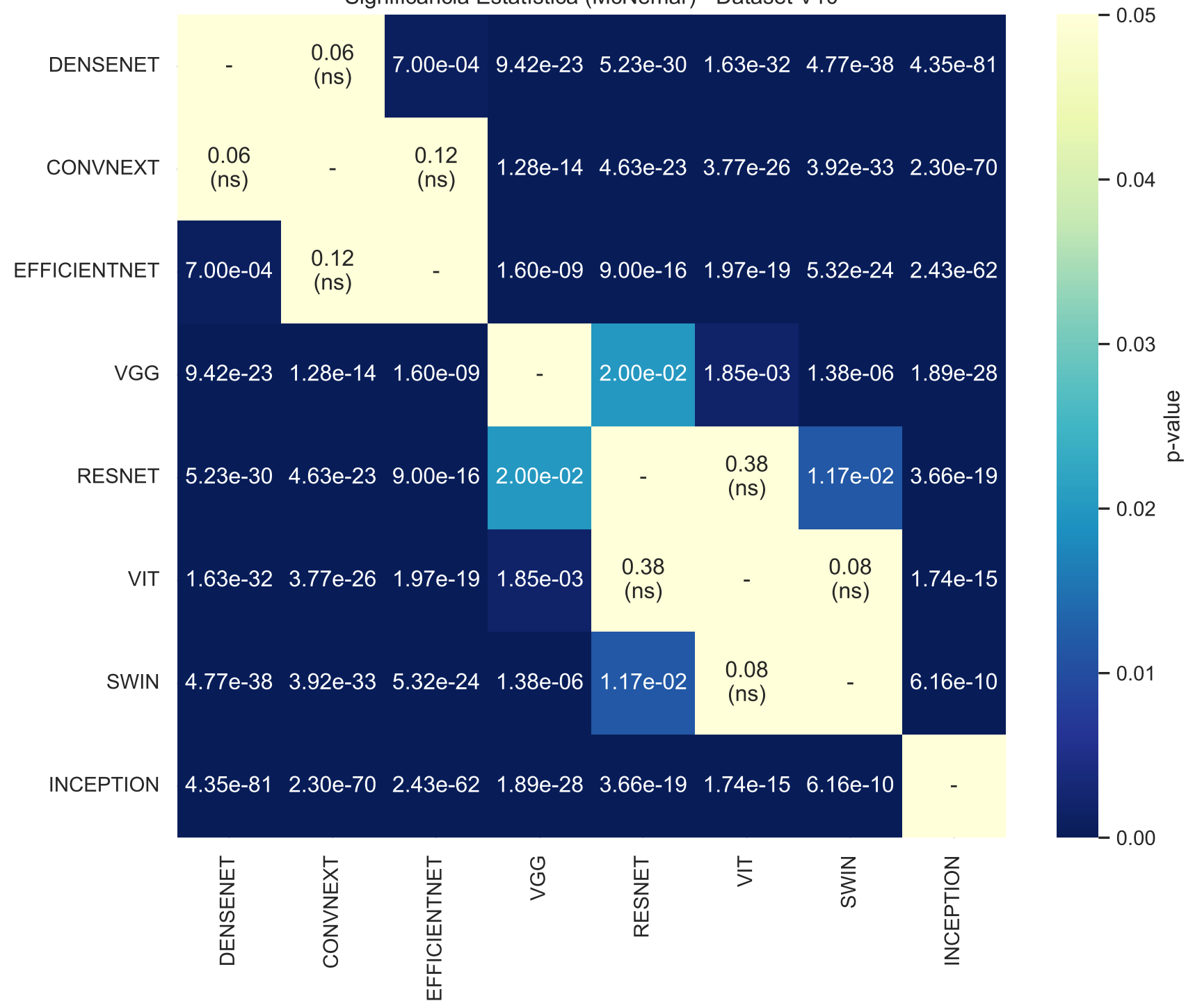
Significância Estatística (McNemar) - Dataset V10
