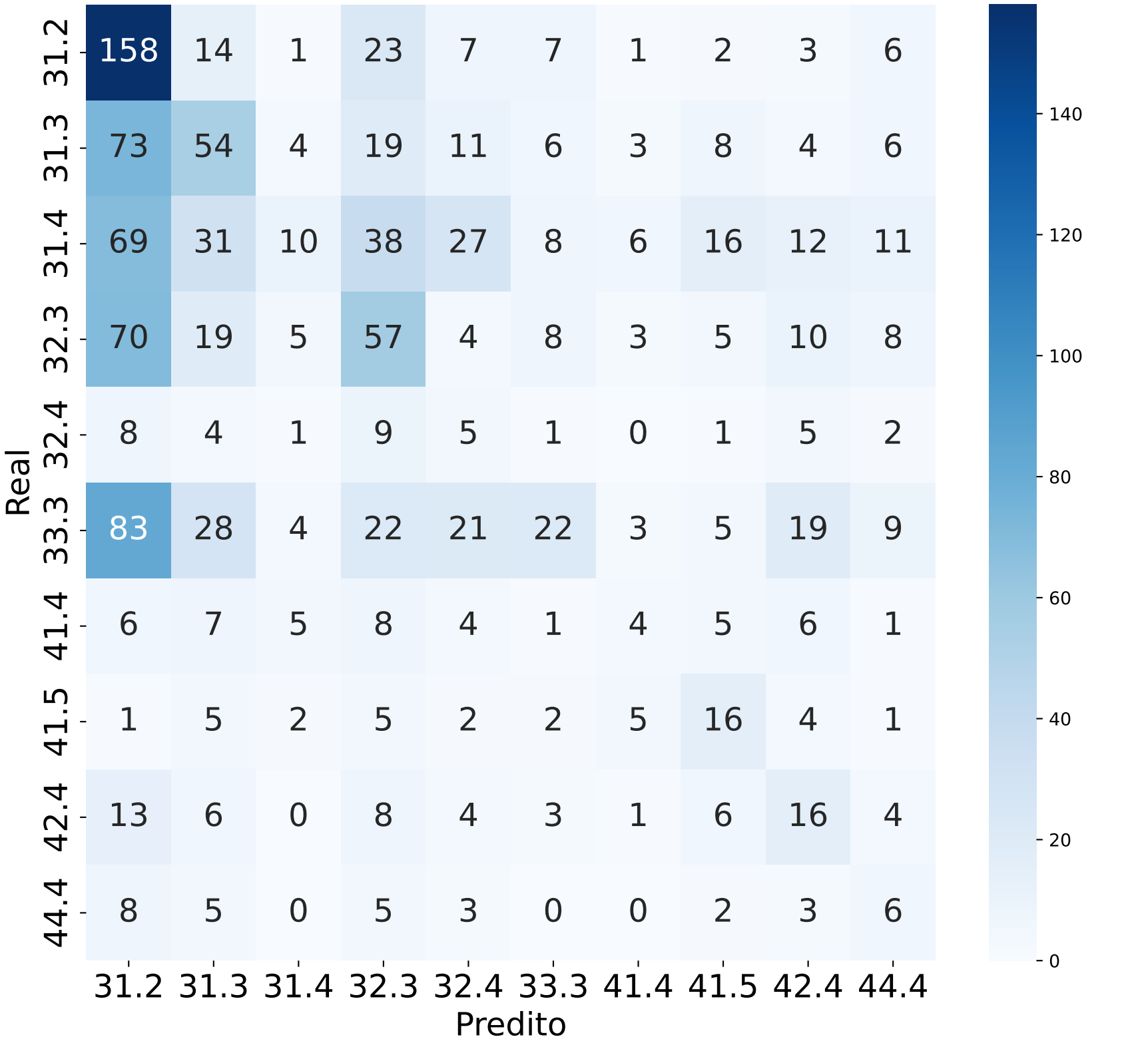
Matriz de Confusão
