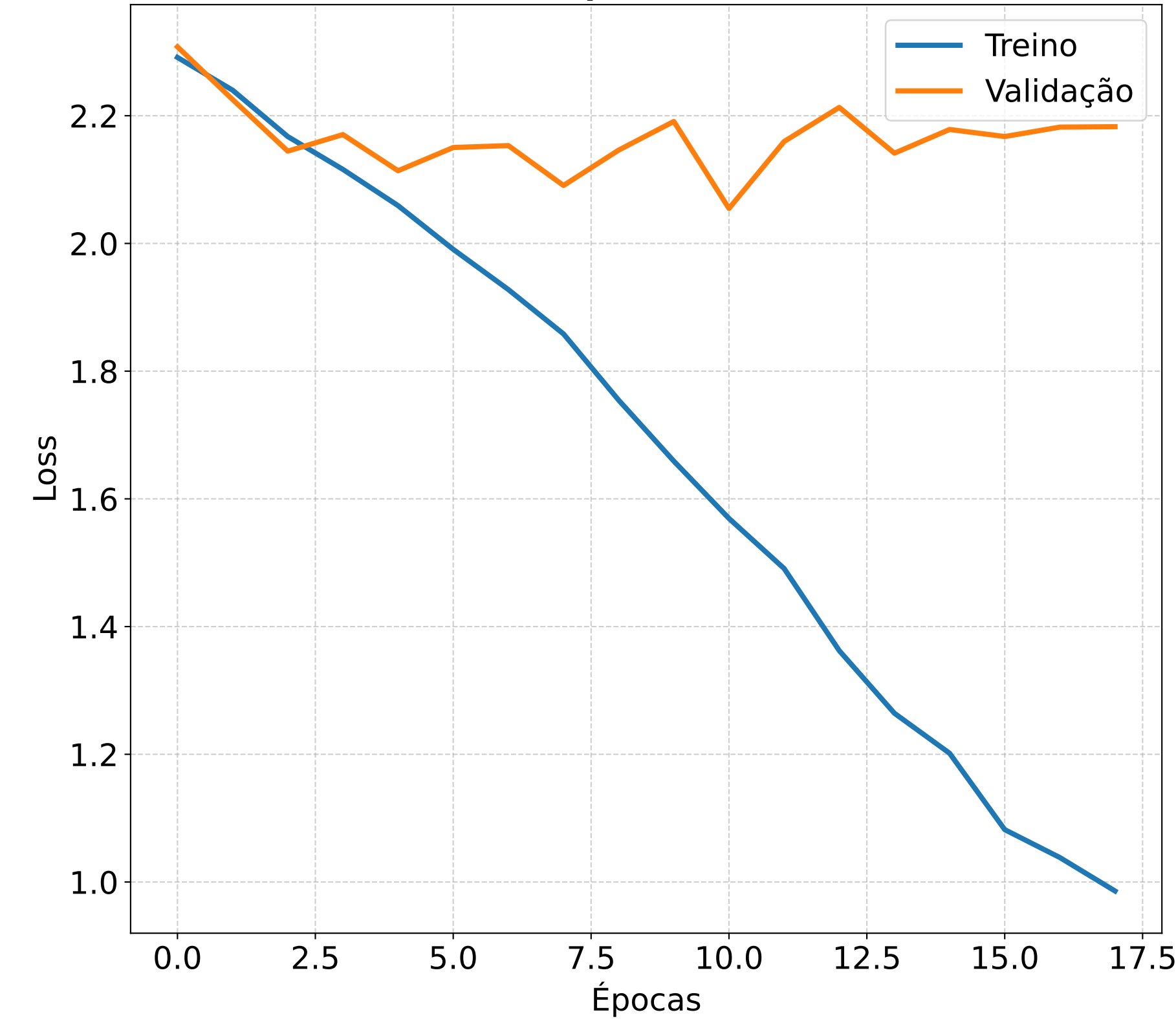
Curva de Aprendizado (Loss)
