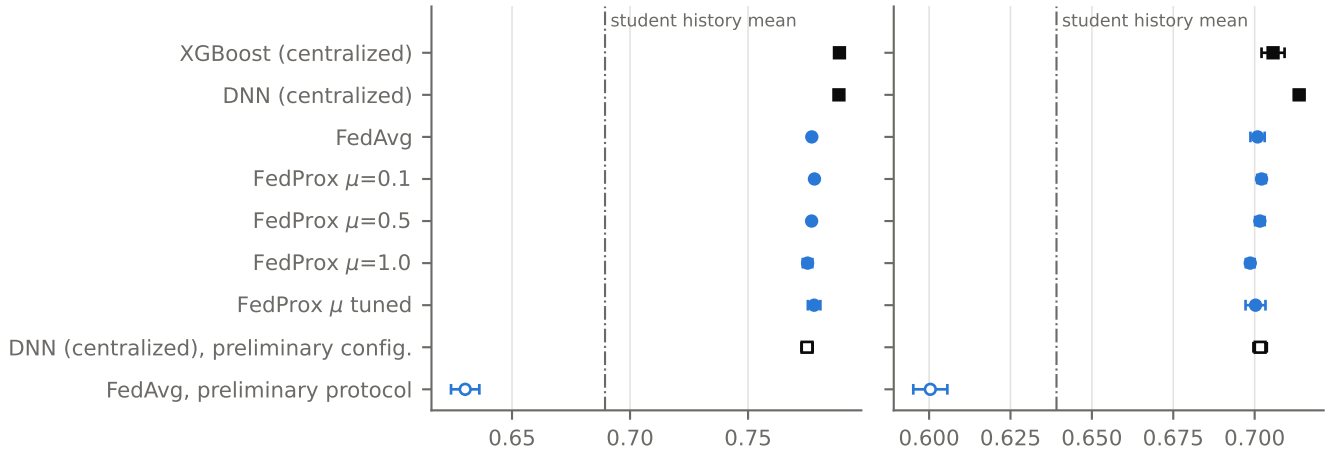
(a) Test ROC AUC
