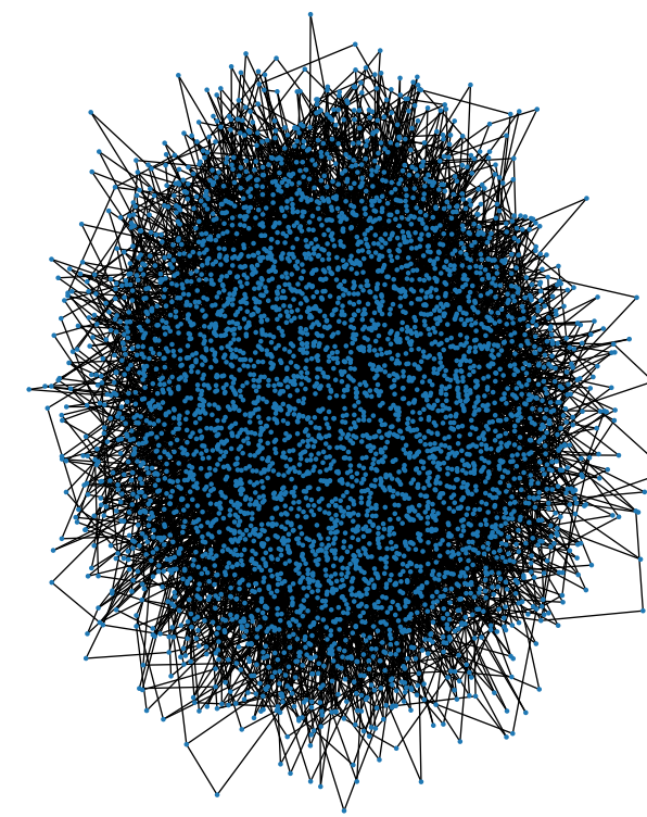
Barabási-Albert
