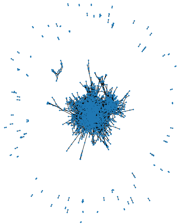
Cora
