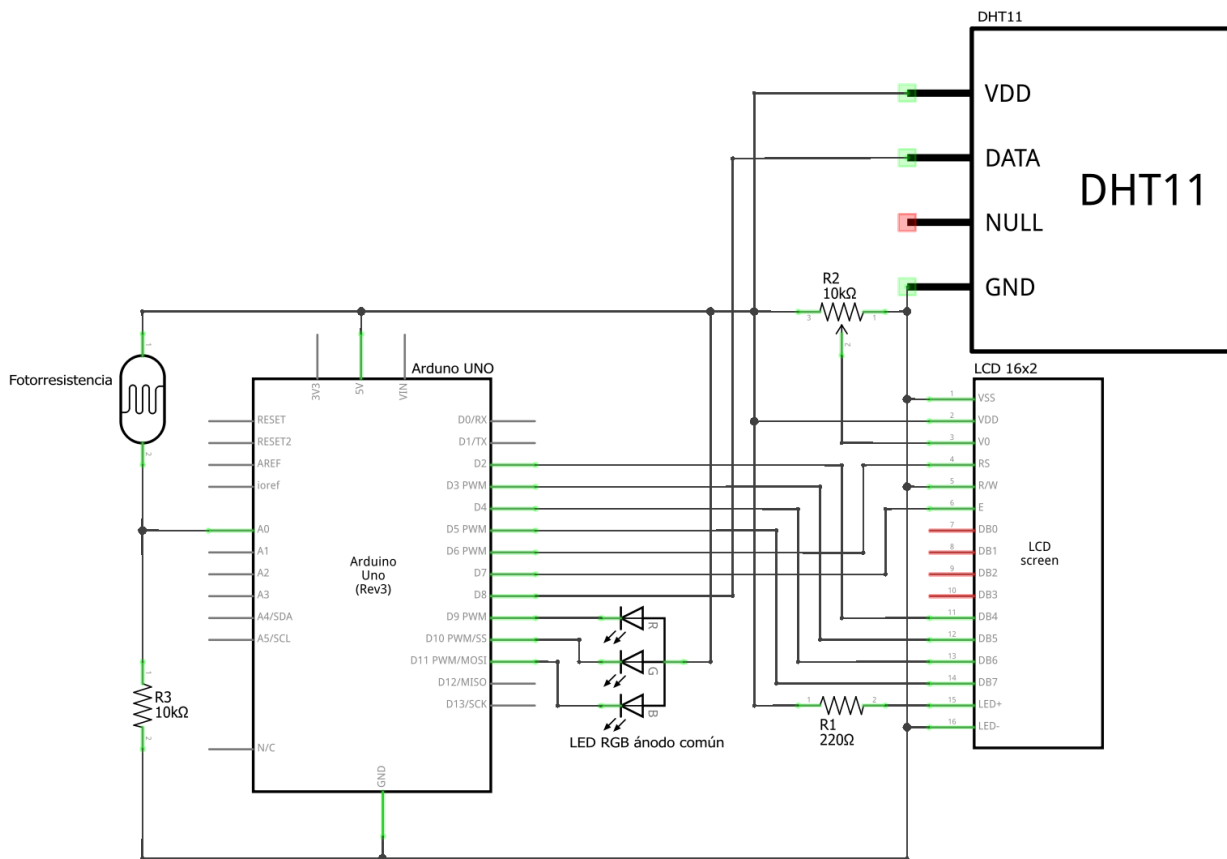
Figura 1: Cicuito con LCD y sensores
