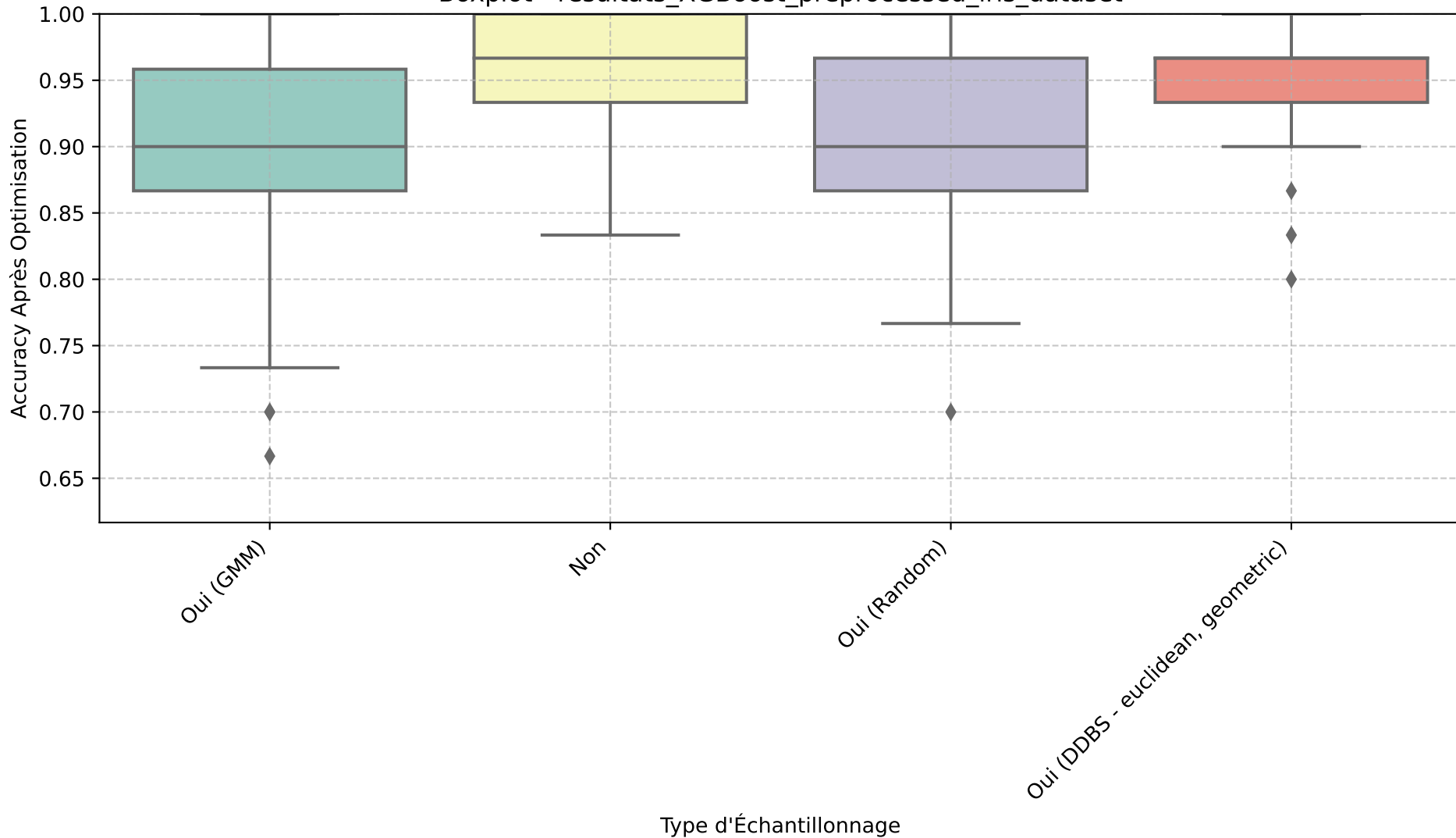
Boxplot - resultats_XGBoost_preprocessed_iris_dataset
