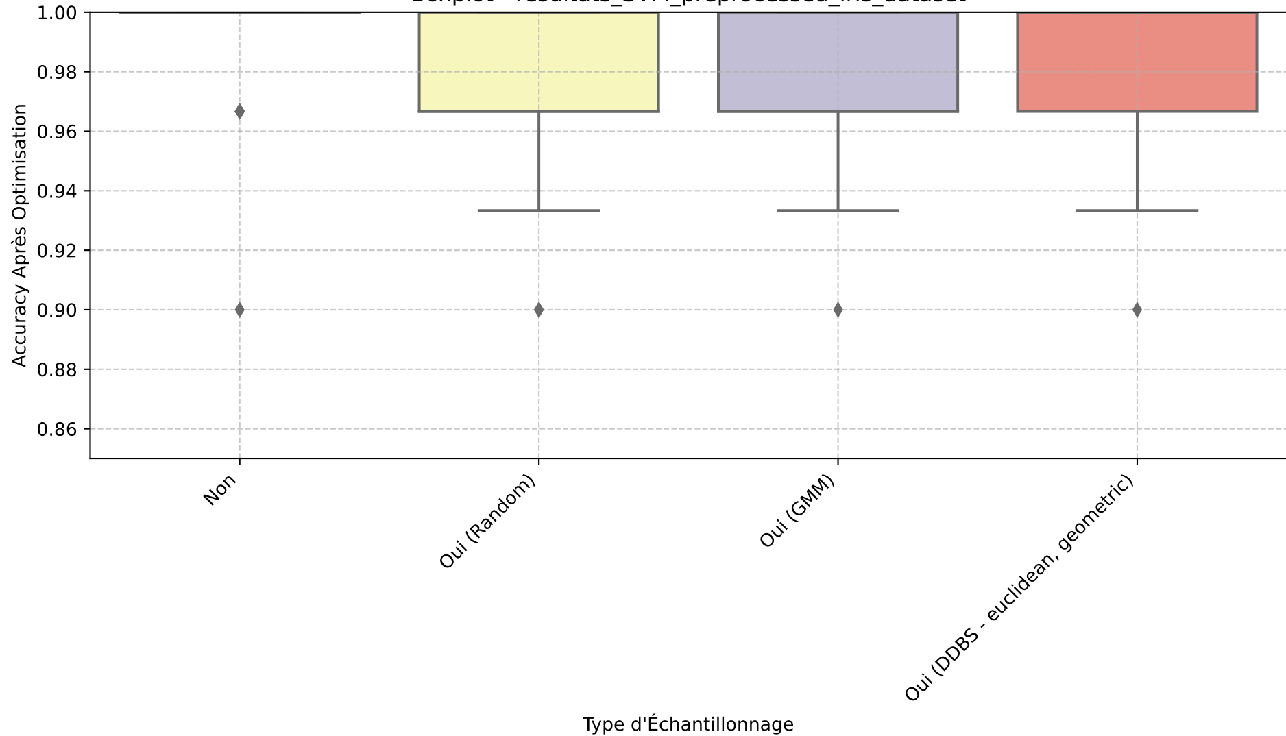
Boxplot - resultats_SVM_preprocessed_iris_dataset
