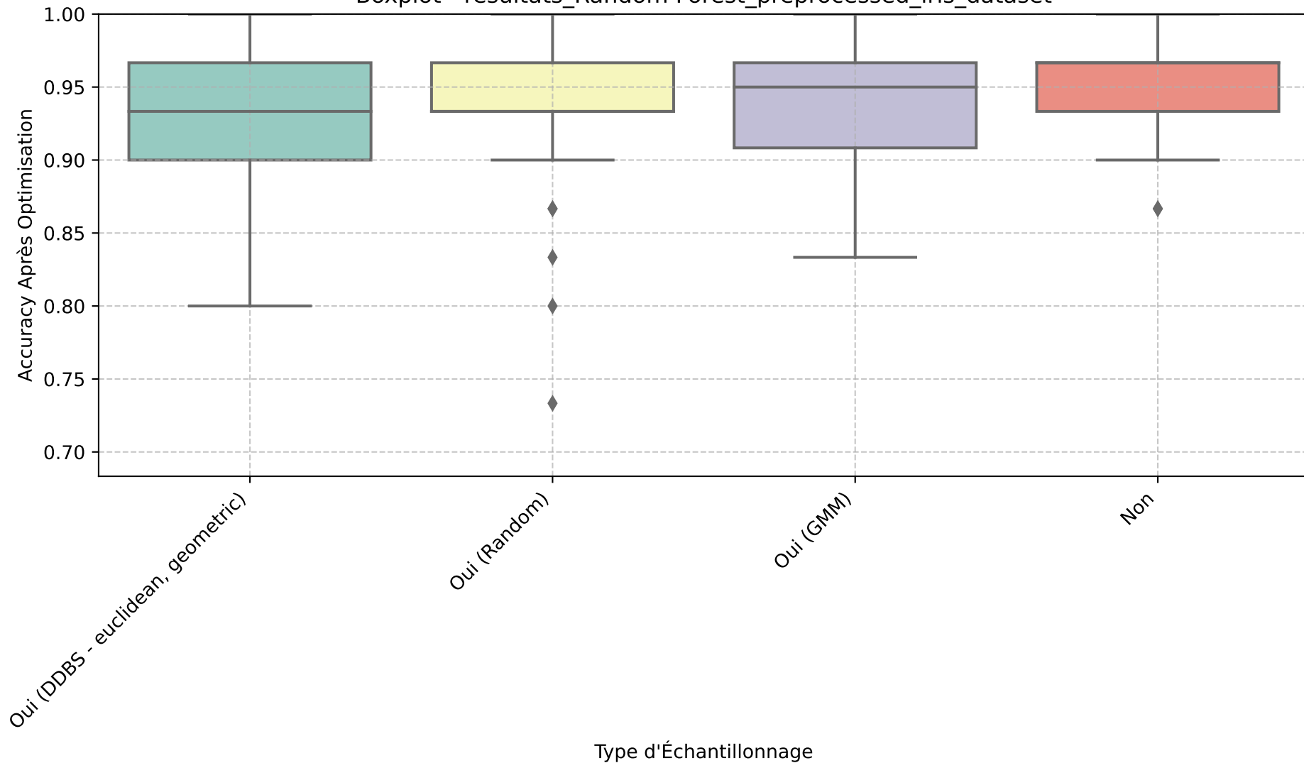
Boxplot - resultats_Random Forest_preprocessed_iris_dataset
