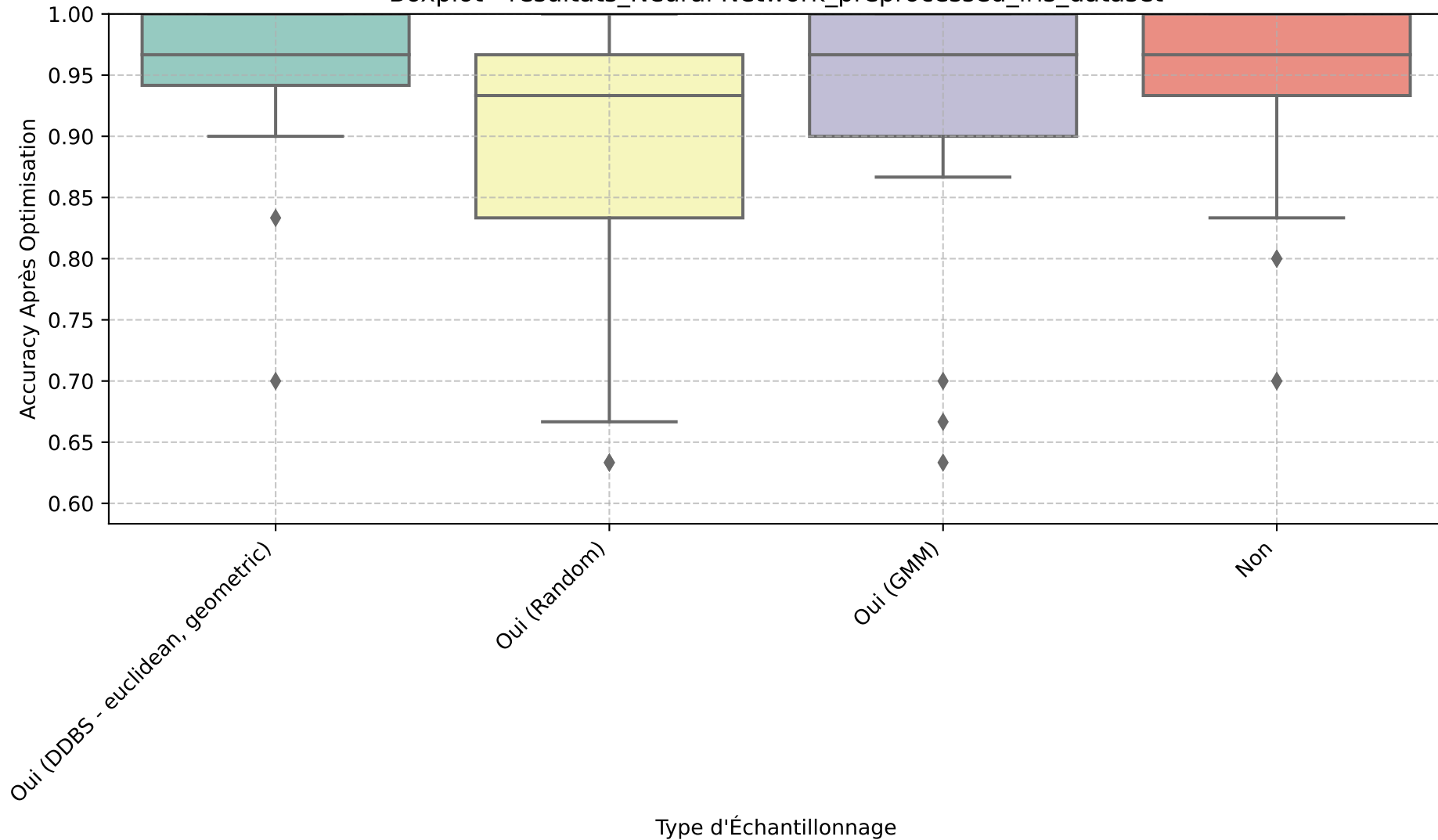
Boxplot - resultats_Neural Network_preprocessed_iris_dataset
