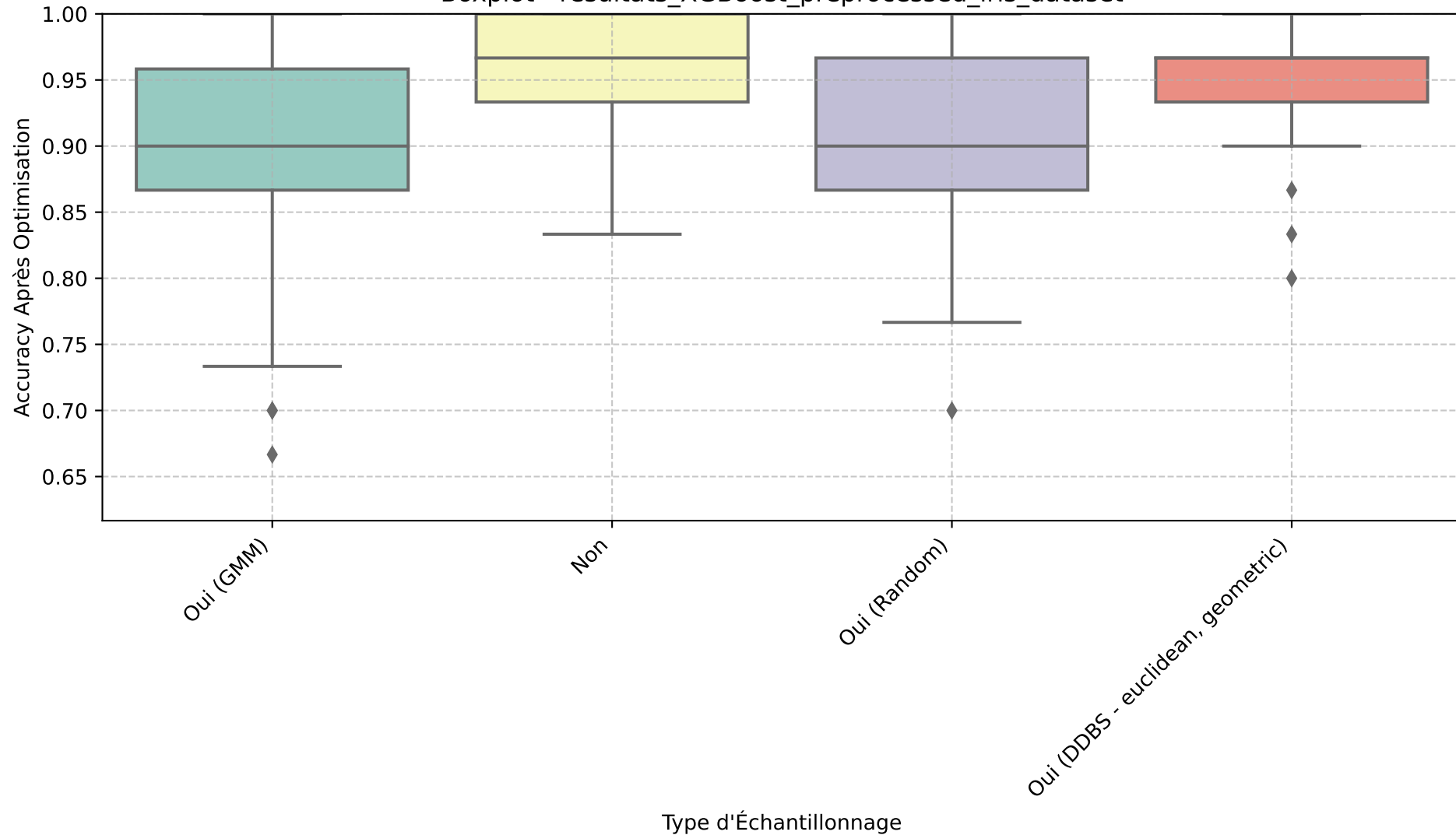
Boxplot - resultats_XGBoost_preprocessed_iris_dataset
