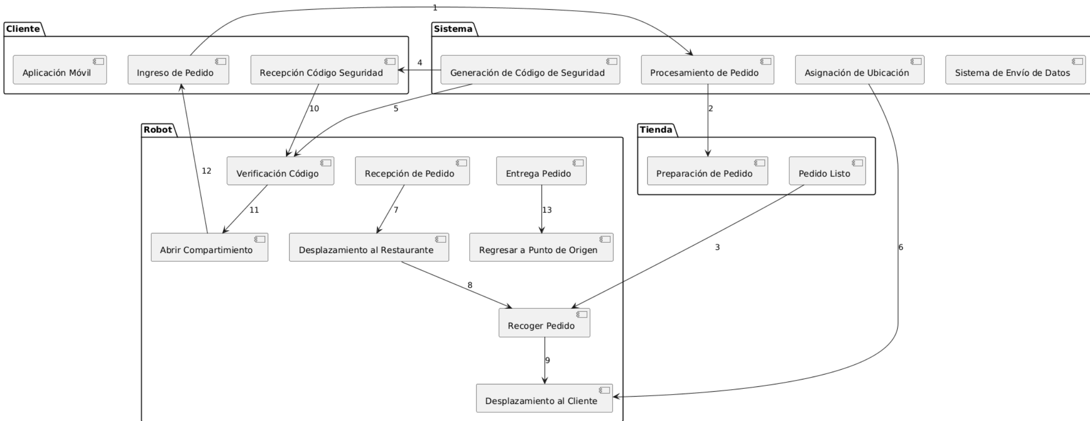
Fig. 1 - Diagrama de bloques del sistema RD2 (Robot Delivery)
