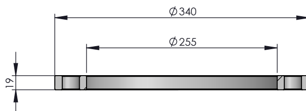
SEÇÃO A-A
